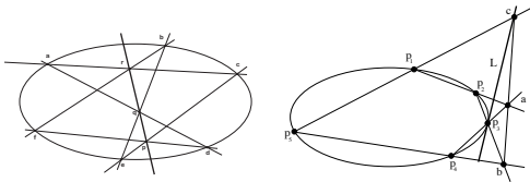
Figure 2: L'hexagramme de Pascal et construction d'une tangente
