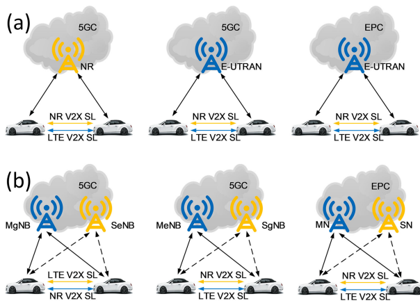
FIGURE 11. NR V2X operation scenarios. (a) V2X SL standalone scenarios, (b) V2X SL MR-DC scenarios [27].
