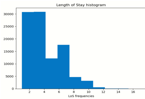
Fig. 3. Histogram of the LoS variable.
