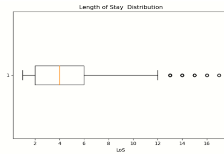
Fig. 4. Boxplot of the LoS variable.
