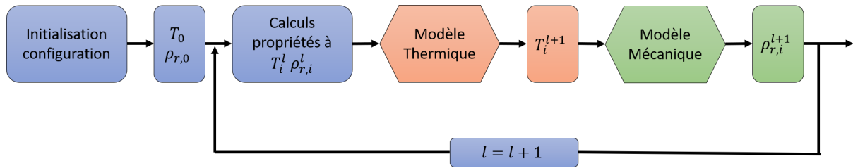
Figure 4 : Schéma du processus du couplage thermomécanique
