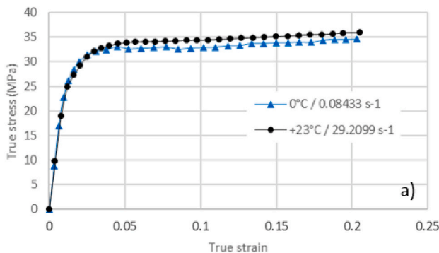
Fig. 13. 2 couples tested a) 0 °C/+23 °C b) +23 °C/+50 °C.
