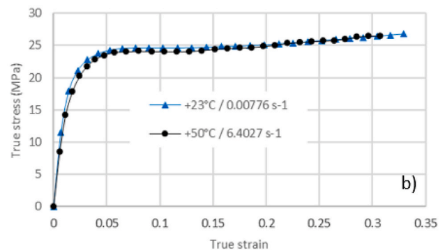
Fig. 13. 2 couples tested a) 0 °C/+23 °C b) +23 °C/+50 °C.
