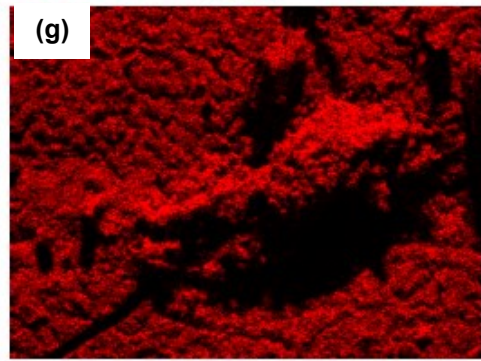
O Kα1
