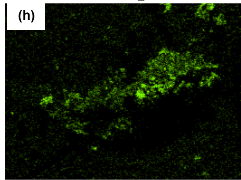
Na Kα1_2
