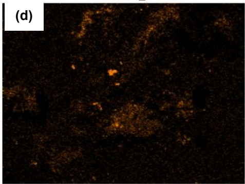
Na Kα1_2
