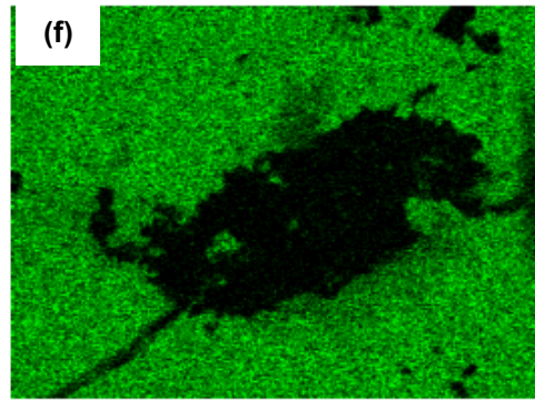
Fe Kα1
