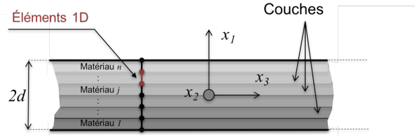
FIGURE 2 – Discrétisation de l'épaisseur d'une plaque multicouche.
