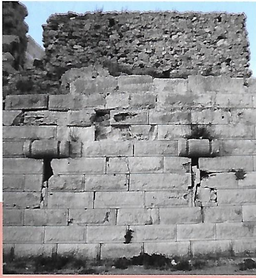
Atış Pencereleri bulunan Hellenistik Surlar Hellenistic fortification with shooting windows
