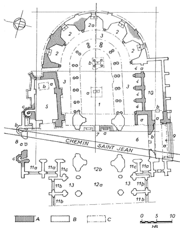
FIG. 2. — Plan de la zone du chœur et du transept de l'ancienne cathédrale de Théroüanne, d'après Honoré Bernard. © L. Dalmau 2016.
