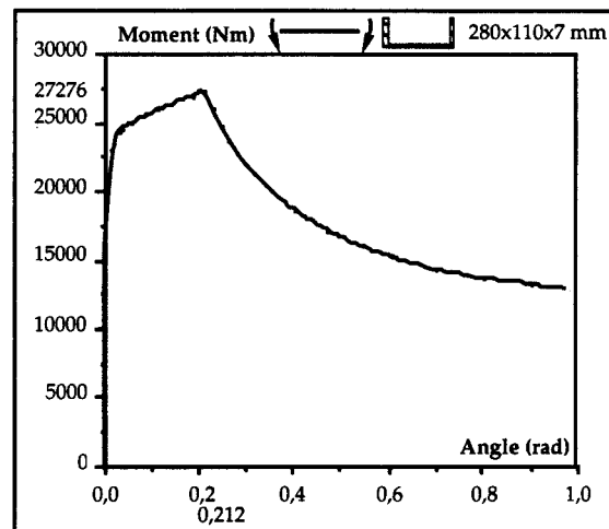
FIG. 5.9a. Longeron droit frontal (élément n° 14).
