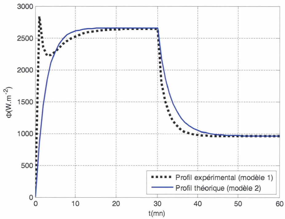
Figure IV.37 : Comparaison du flux pariétal pour U_\infty=5 m/s (vitrocéramique)
