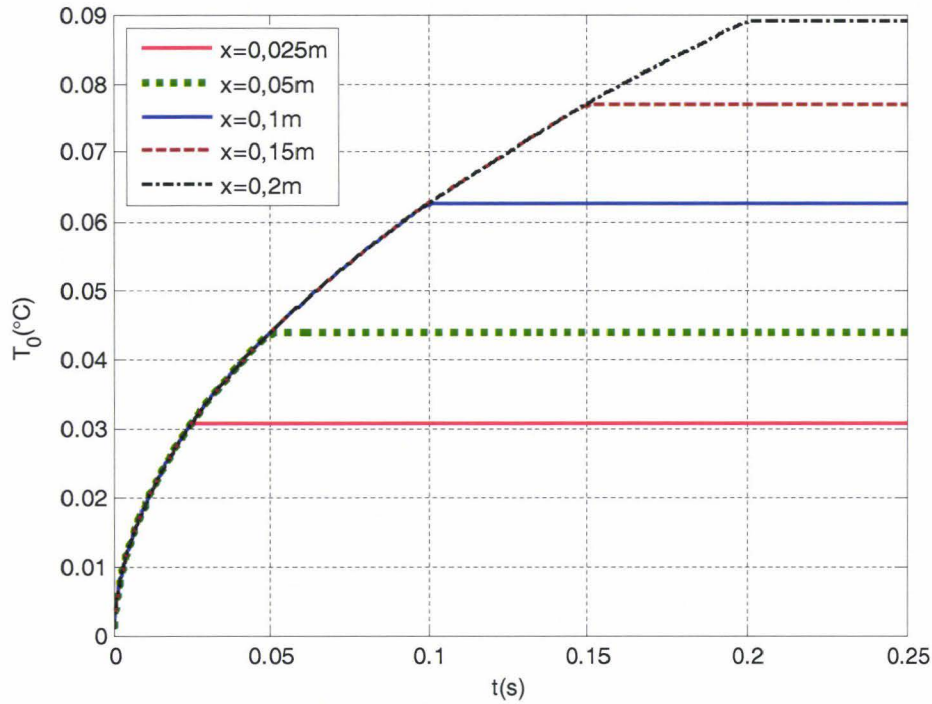
Figure III.6 : Evolution temporelle de la température pariétale T_0 pour différents x
