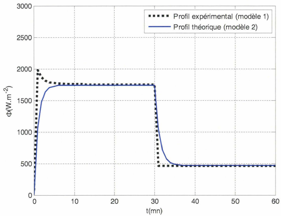
Figure IV.39 : Comparaison du flux pariétal pour U_\infty=5 m/s (Aluminium)
