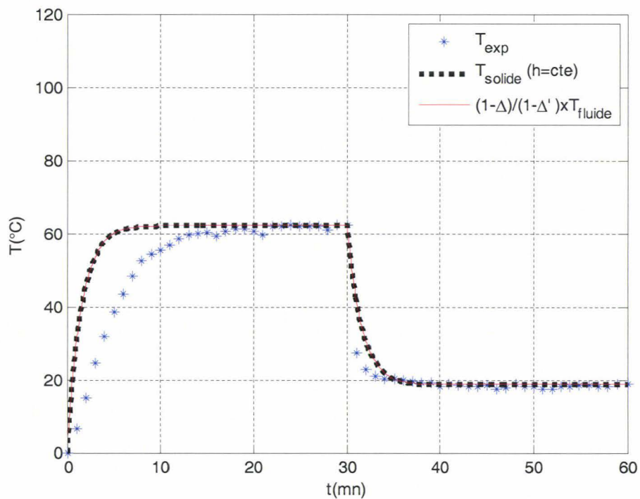
Figure IV.35 : Comparaison des profils de température pour une vitesse d'écoulement 5 m/s (Aluminium)
