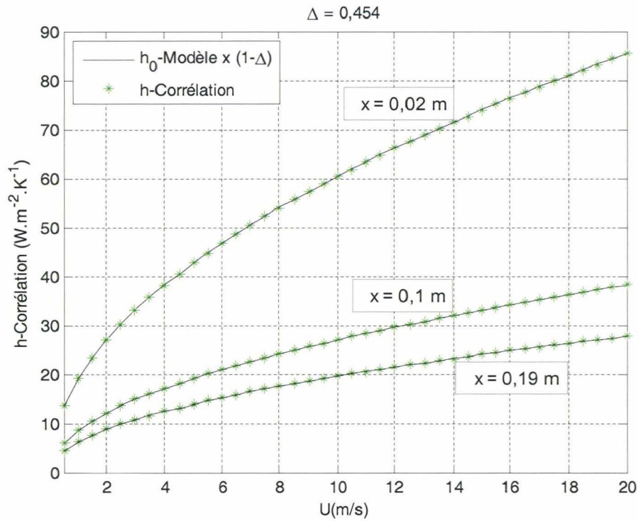
Figure III.18 : Comparaison du h_0(x) du modèle et de la corrélation ( 0,5 < U_\infty < 20 \text{ m/s} )
