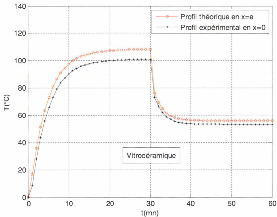
Figure IV.15 : Profil de température pour U_{\infty} = 7 m/s (modèle 1)
