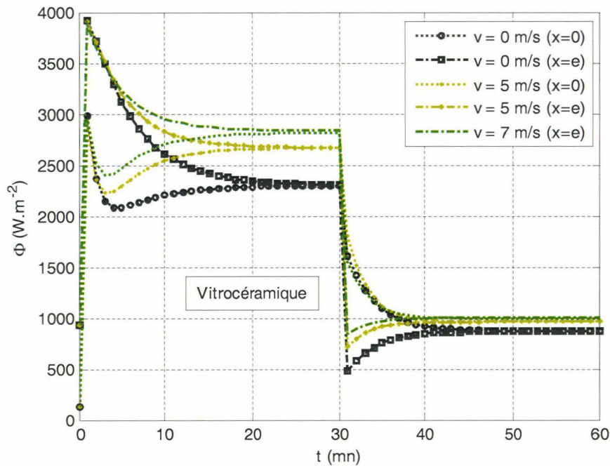
Figure IV.17 : Flux de chaleur pariétaux pour différentes vitesses d'écoulement
