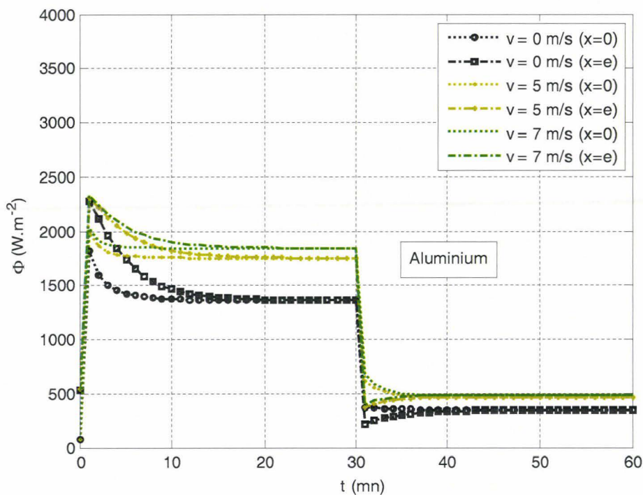
Figure IV.18 : Flux de chaleur pariétaux pour différentes vitesses d'écoulement
