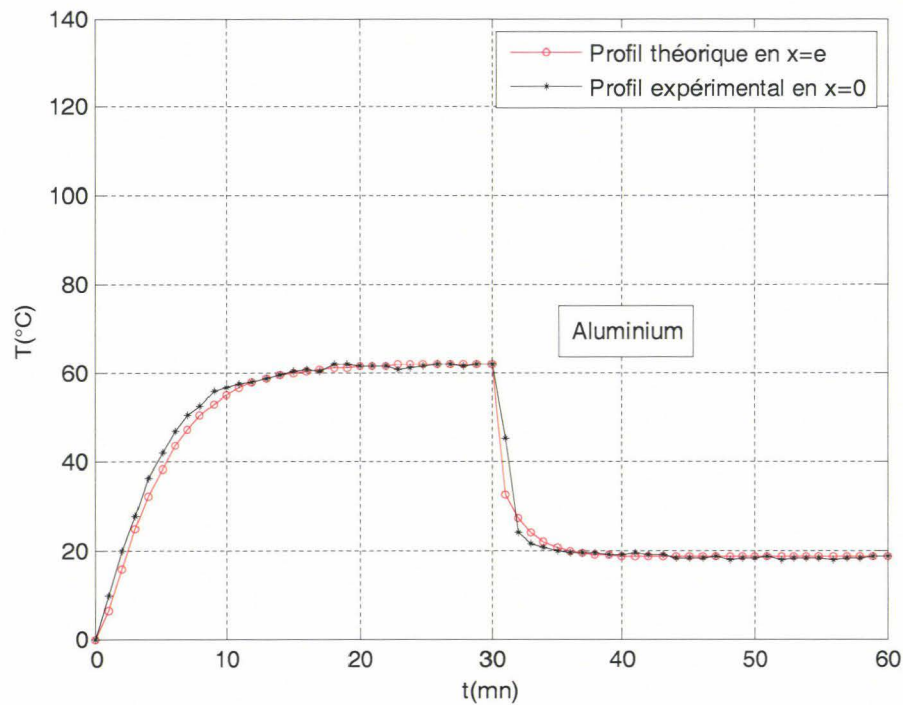
Figure IV.14 : Profil de température pour U_{\infty} = 5 m/s (modèle 1)
