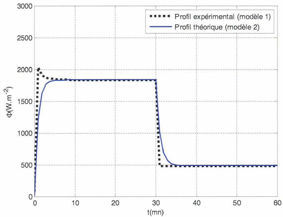
Figure IV.40 : Comparaison du flux pariétal pour U_\infty=7 m/s (Aluminium)
