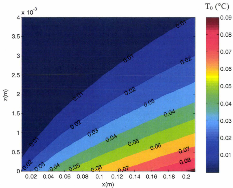
Figure III.16 : Couche limite thermique en régime permanent
