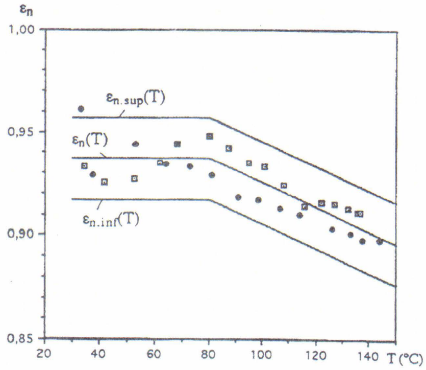
Figure.1 : Variation de l'émissivité \epsilon_n de la peinture noire avec la température
