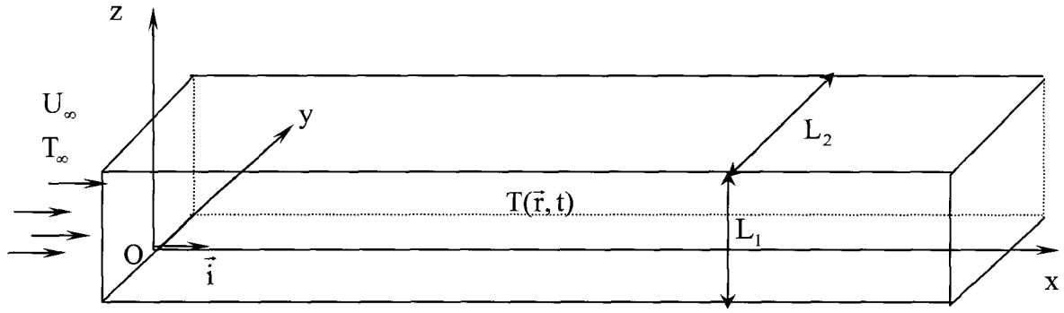
Figure III.1 : Représentation de l'écoulement dans un canal rectangulaire
