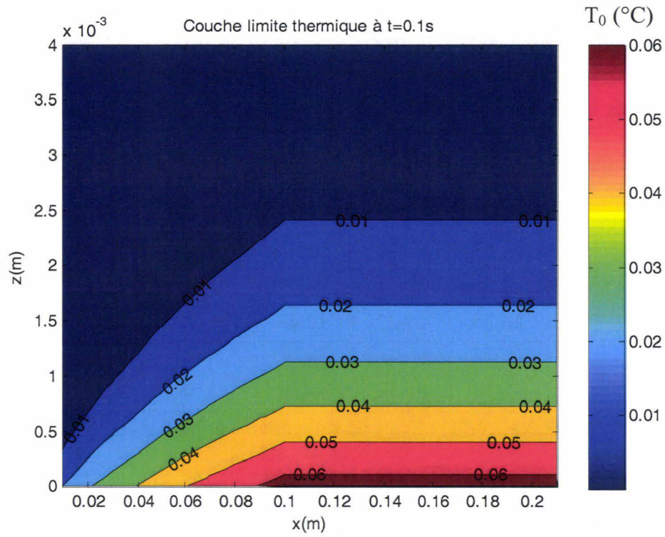
Figure III.15 : Couche limite thermique en régime transitoire
