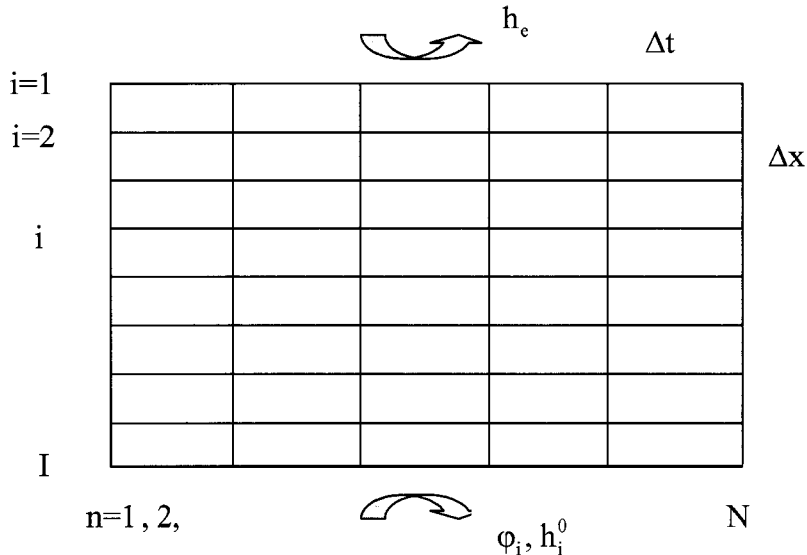
Figure 1 : Discrétisation de la plaque par différences finies
