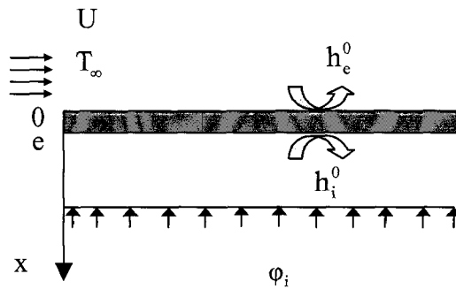
Figure IV.10 : Représentation schématique des conditions aux limites sur la plaque au régime permanent
