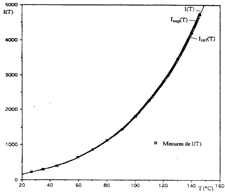
Figure.2 : Variation des mesures du signal de sortie de la caméra en fonction de la température du corps noir
