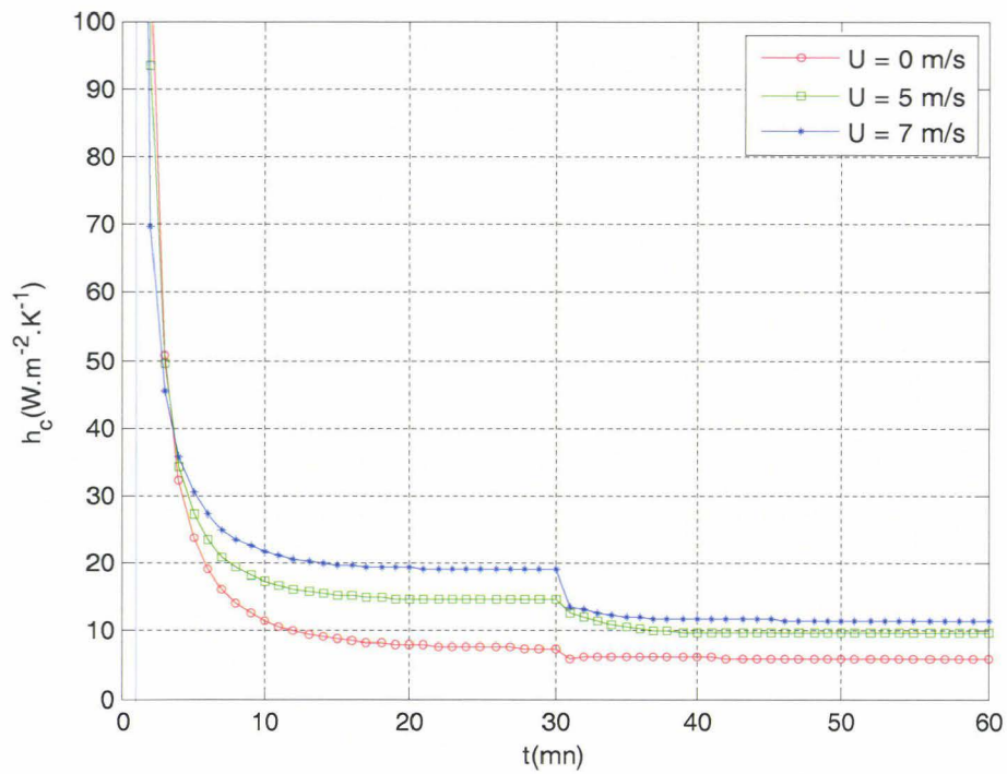
Figure IV.22 : Coefficients d'échanges convectifs pour différentes vitesses d'écoulement (Vitrocéramique)
