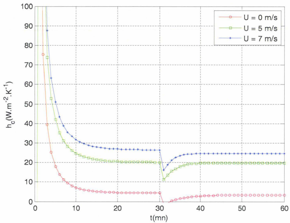
Figure IV.23 : Coefficients d'échanges convectifs pour différentes vitesses d'écoulement (Aluminium)
