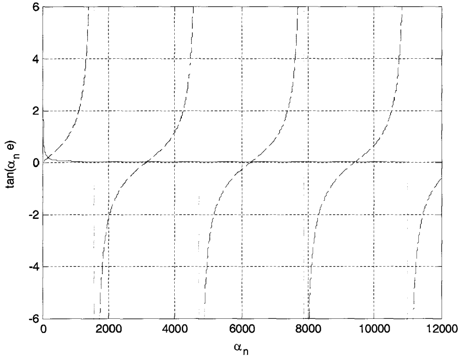
Figure II.3 : Valeurs propres du Laplacien
