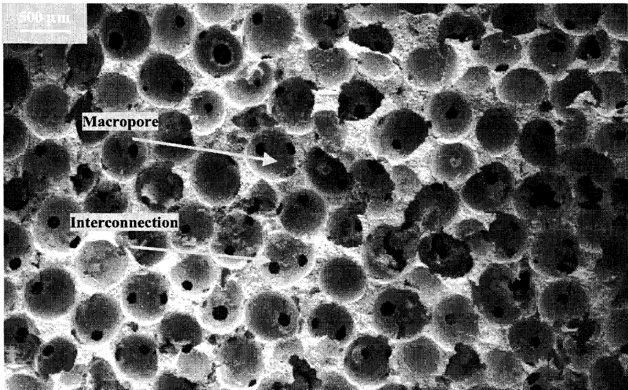
Figure 43 : Observation MEB d'une structure macroporeuse issue du verre P3C2 après déliantage.
