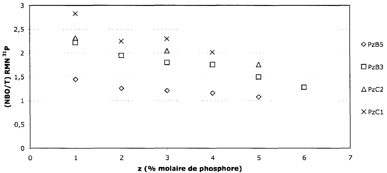
Figure 33 : Evolution du rapport NBO/T calculé à partir des données de la RMN du 31 P, en fonction du taux de P 2 O 5 introduit dans les verres, pour les séries PzB5, PzB3, PzC2 et PzC1
