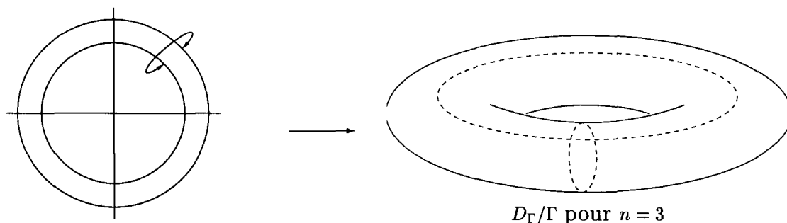
Action de \Gamma sur D_\Gamma pour n = 3
