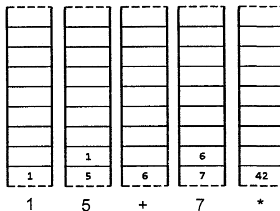
Figure 70 – Exemple d'utilisation de la pile en FORTH . Nous noterons la forte ressemblance avec la notation polonaise inversée, notamment utilisée par le langage de description de page PostScript ou par les calculateurs signés Hewlett-Packard .
