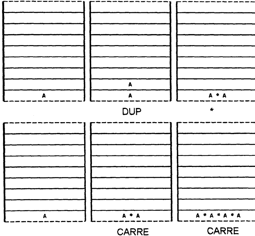
Figure 71 – Résultat sur la pile de l'exécution des mots CARRE (haut de la figure) et PUISSANCE4 (bas de la figure).
