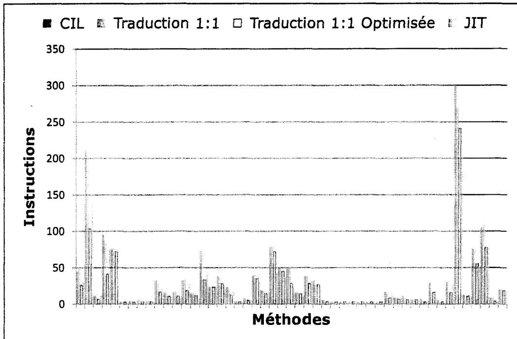
Figure 51 – Nombre d'instructions générées pour XMLMark 1.1.
