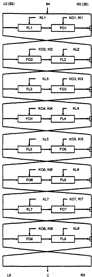
Figure 40 – Algorithme de Kasumi – Source : 3GPP. ⊕ représente un ou exclusif. FOx et FLx sont des sous-fonctions de Kasumi. Chaque sous-fonction utilise des clés pour encoder les données.
