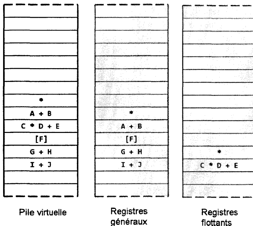
Figure 36 – État final de la pile virtuelle. * représente xtos.
