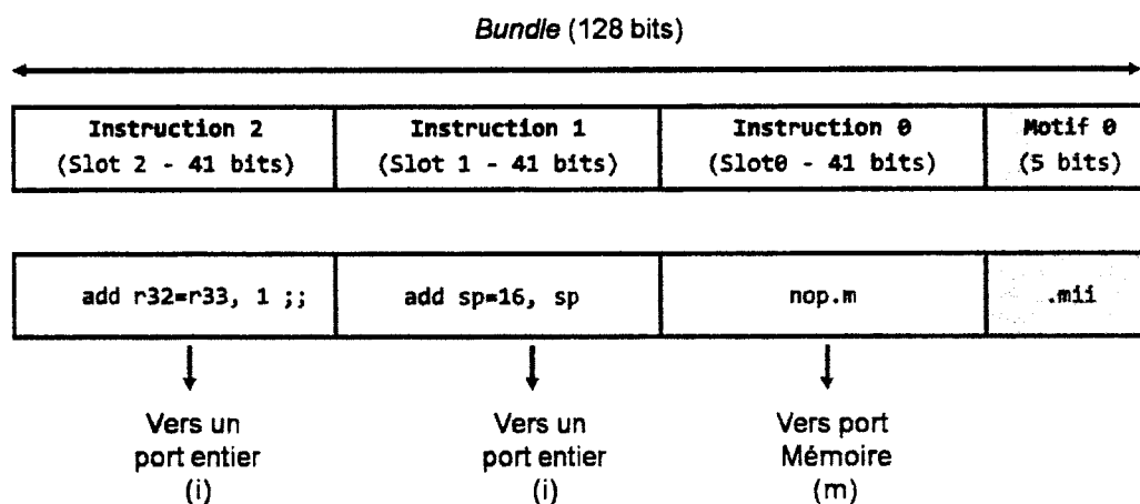
Figure 68 – Format d'une instruction de processeur Itanium .
