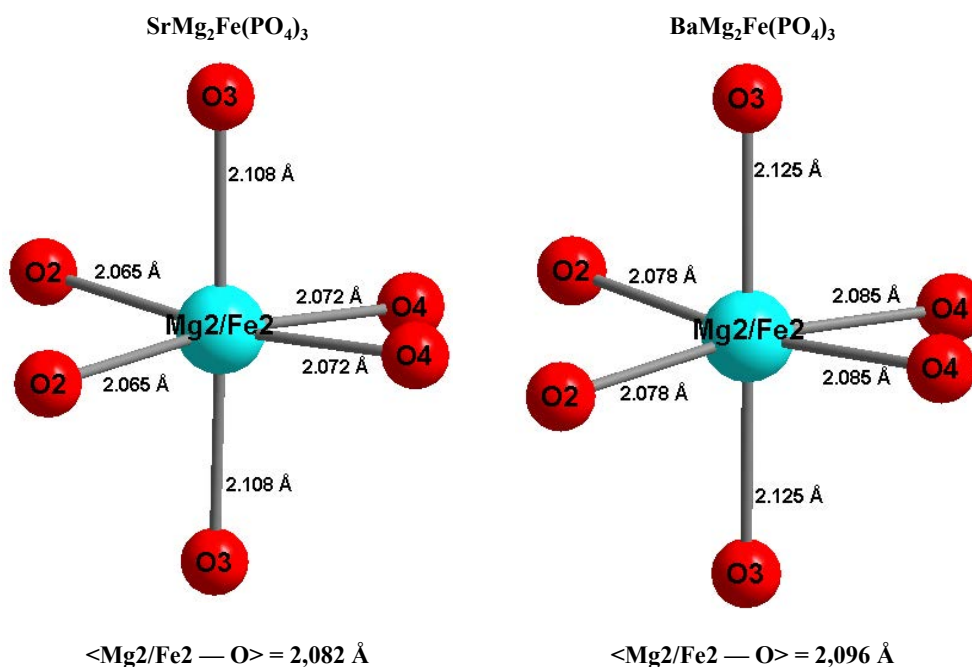
Figure III-3 : Environnement des ions \text{Fe}^{3+} et \text{Mg}^{2+} dans le site Mg2/Fe2 pour les composés \text{MMg}_2\text{Fe}(\text{PO}_4)_3 ( \text{M} = \text{Sr}, \text{Ba} )
