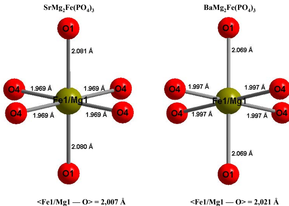
Figure III-2 : Environnement des ions \text{Fe}^{3+} et \text{Mg}^{2+} dans le site Fe1/Mg1 pour les composés \text{MMg}_2\text{Fe}(\text{PO}_4)_3 ( \text{M} = \text{Sr}, \text{Ba} )
