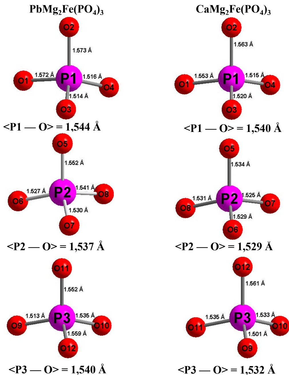
Figure III-12 : Environnement de l'ion \text{P}^{5+} dans les sites P1, P2 et P3 pour les composés \text{MMg}_2\text{Fe}(\text{PO}_4)_3 ( \text{M} = \text{Ca}, \text{Pb} )
