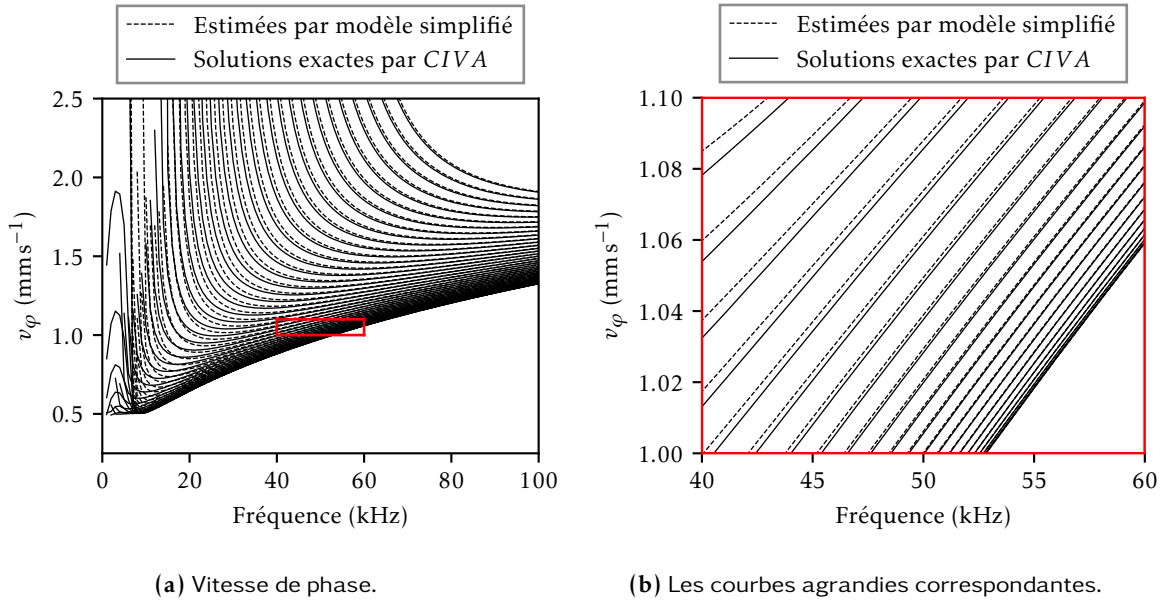
FIGURE 1.8 – Courbes de dispersion pour la famille de modes (longitudinal) antisymétrique-flexions F(n,1) d'un tube en acier inoxydable de 2,145 mm d'épaisseur calculées par le modèle simplifié et par CIV A.
