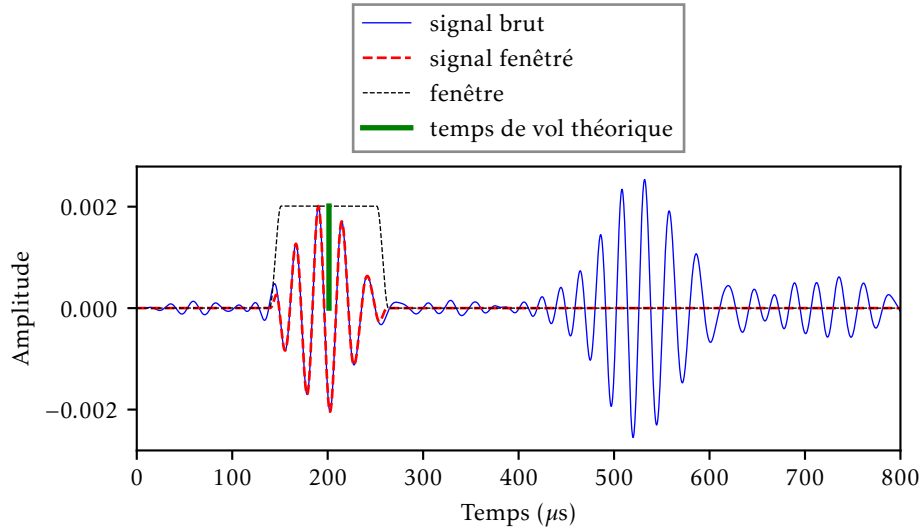
FIGURE 3.9 – Exemple de signal simulé fenêtré pour obtenir la partie utile du signal. Le temps de vol théorique de la famille de mode L(0,1) utilisé pour choisir la fenêtré est aussi présenté.
