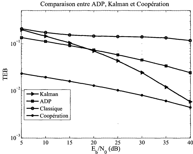
FIGURE 4.11 – Comparaison entre les estimations du canal pour QPSK.
