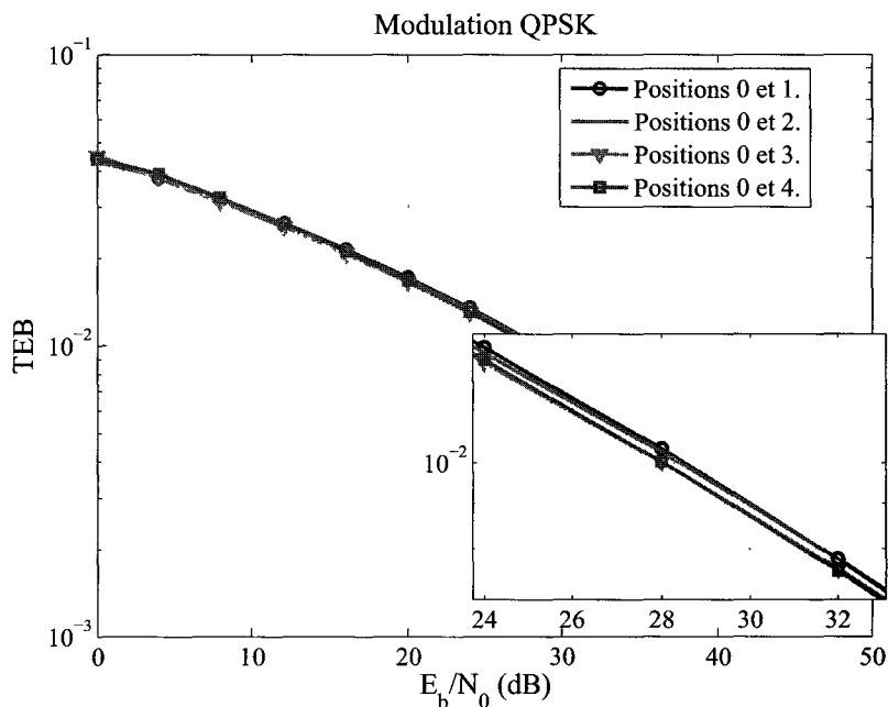
FIGURE 4.14 – Effet des positions des sous-porteuses pilotes, cas de deux utilisateurs.
