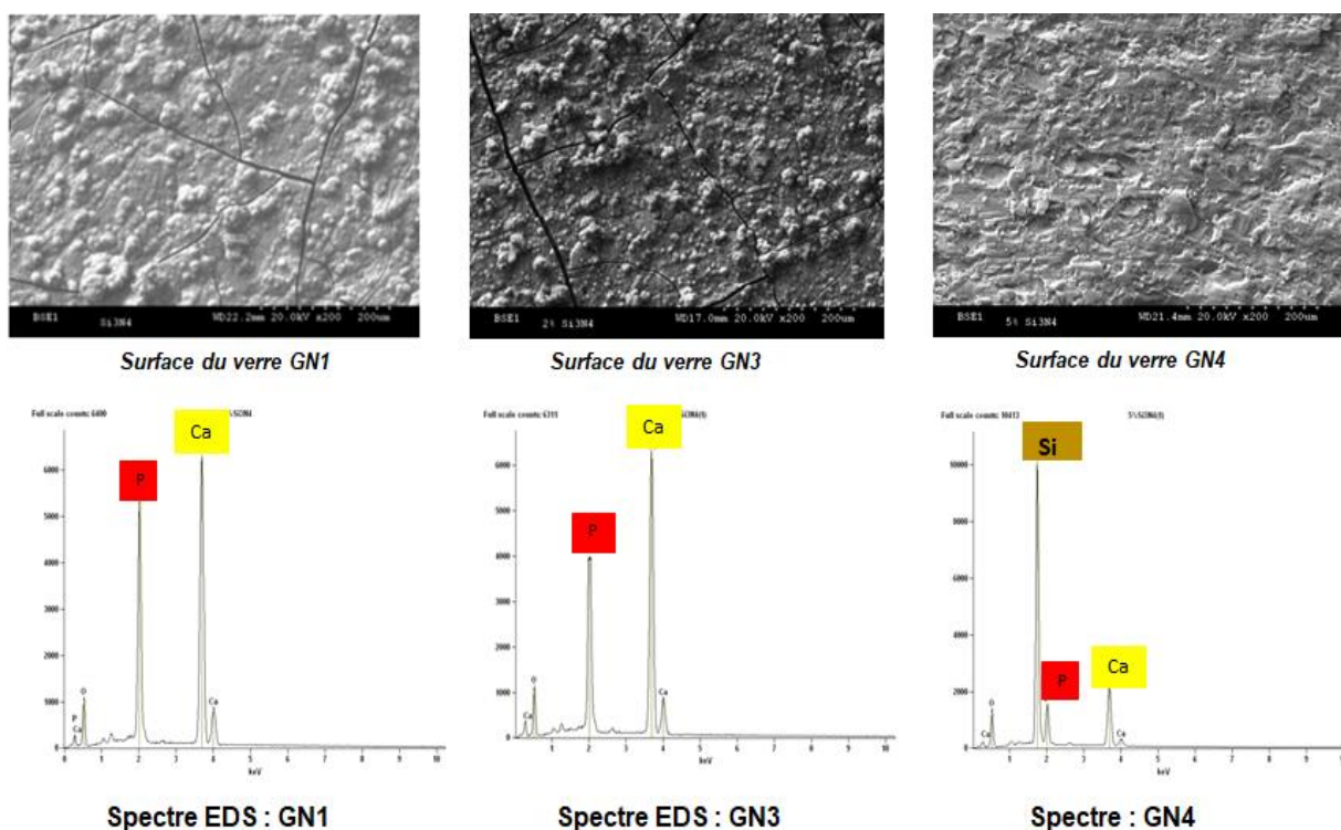
Figure 25 : spectres EDS et photos MEB des surfaces des verres oxynitridés GNx après 15 jours d'immersion dans le SBF.
