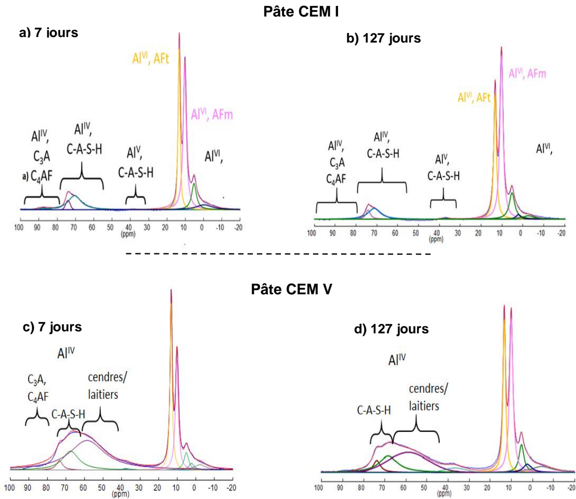
Figure 81 : décompositions des spectres RMN-MAS- ^{27}\text{Al} (18,8 T) des pâtes sans piègeur a) CEM I à 7 jours, b) CEM I à 127 jours, c) CEM V à 7 jours et d) CEM V à 127 jours. Spectre expérimental en bleu, spectre simulé en rouge.
