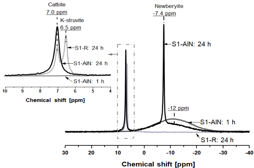
Figure 74 : spectres RMN MAS ^{31}P (9,4 T) avec découplage proton des pâtes de ciment S1-R et S1-AIN en fonction du temps d'hydratation.
