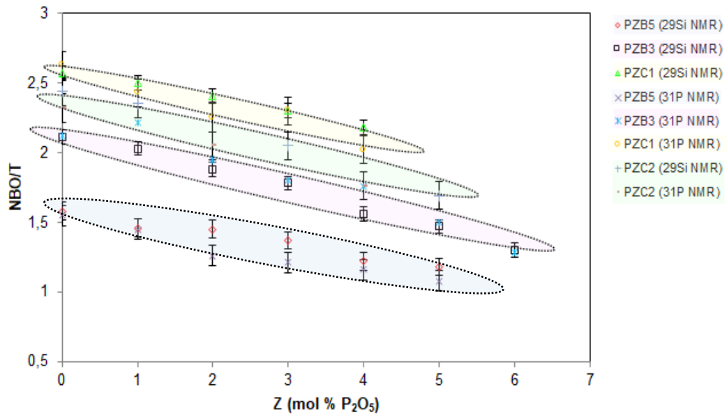
Figure 10 : évolution des valeurs NBO/T déterminées par RMN 29 Si et du 31 P en fonction de z % P 2 O 5 des quatre série de verre.
