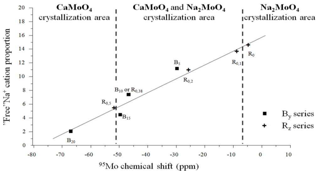
Figure 44 : évolution de la quantité de Na^+ libre en fonction du déplacement chimique du ^{95}Mo dans les verres des séries B_y et R_z .
