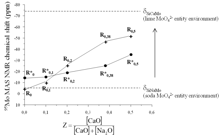
Figure 40 : Variation du déplacement chimique du ^{95}\text{Mo} en fonction du rapport z = \frac{[\text{CaO}]}{[\text{CaO}] + [\text{Na}_2\text{O}]} des verres des séries Rz et Rz^* . Les déplacements chimiques du Mo des verres étalons \text{SiCaMo} et \text{SiNaMo} ont également été reportés et sont représentés par les droites horizontales en pointillés
