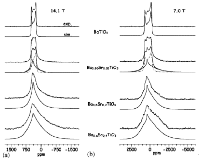
Figure 98 : spectres RMN ^{137}\text{Ba} en statique a) à 14,1 T et b) 7,0 T de \text{Ba}_x\text{Sr}_{1-x}\text{TiO}_3 (ref) à température ambiante [Gervais et al. 2004]
