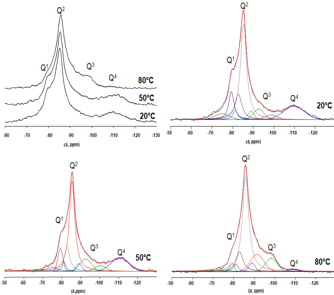
Figure 51 : spectres RMN-MAS du ^{29}\text{Si} (9,4 T) de la pâte B40 hydratée à 6 mois en fonction de la température de cure avec ses décompositions - Spectre expérimental en bleu, spectre simulé en rouge.
