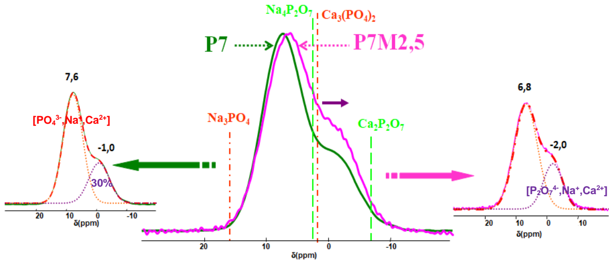
Figure 33 : spectres RMN MAS ^{31}\text{P} (9,4 T) des verres P7 et P7.5 et ses décompositions.
