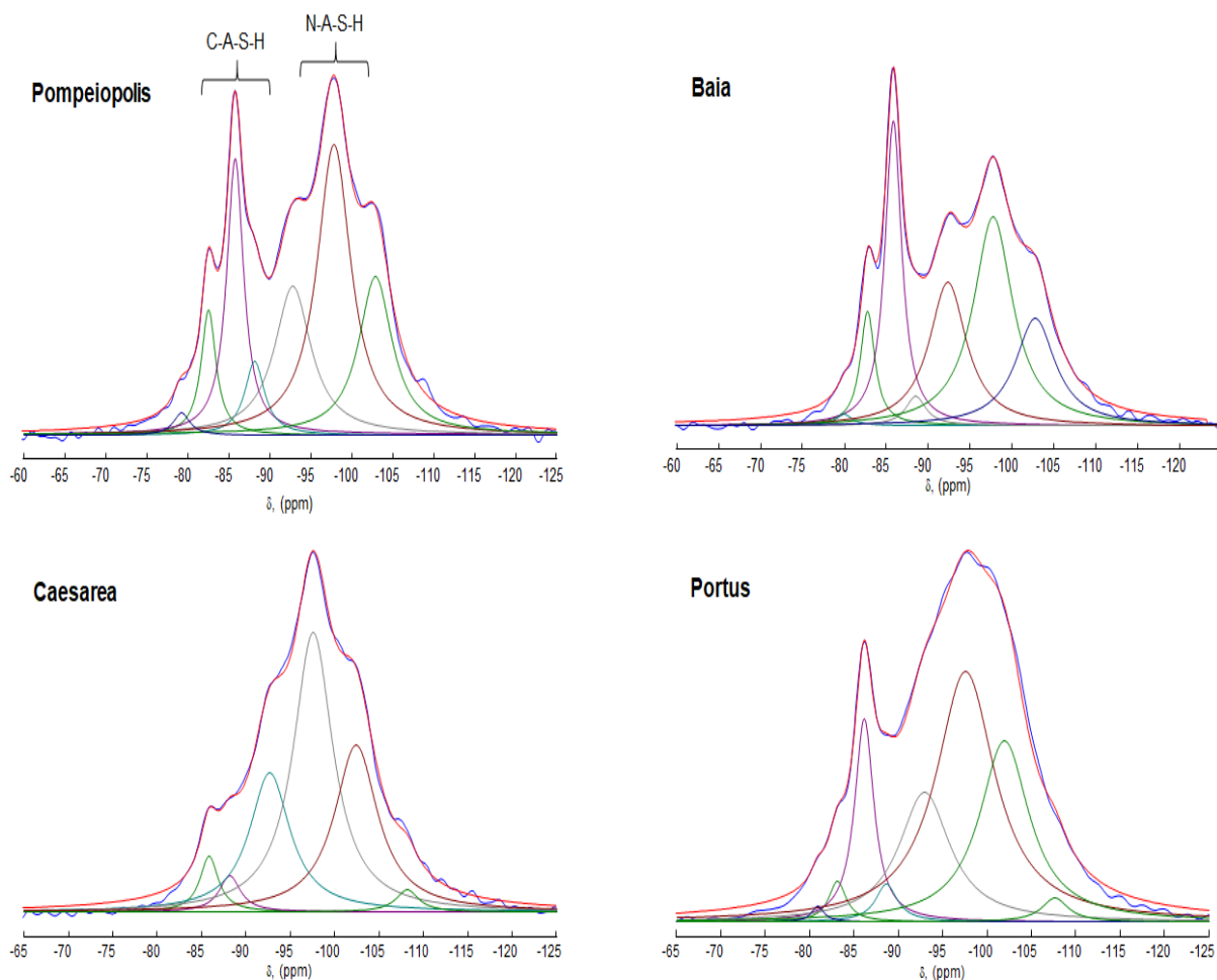
Figure 92 : décompositions des spectres RMN 29 Si des différents bétons romains.
