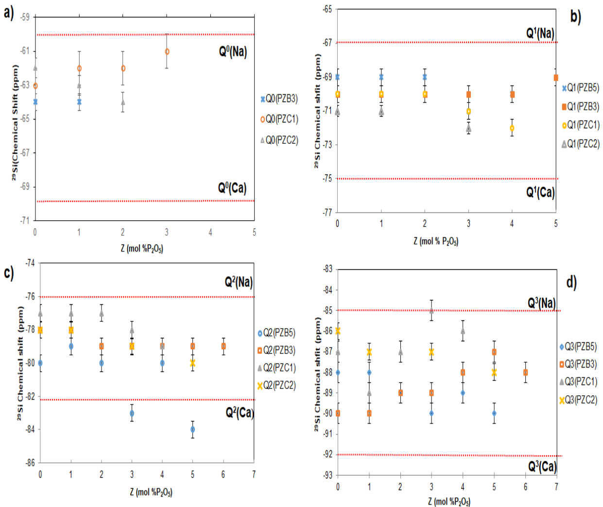
Figure 5 : évolution des déplacements chimiques du Si des entités silicates Q^n a) Q^0 b) Q^1 , c) Q^2 et d) Q^3 en fonction du taux de \text{P}_2\text{O}_5 – Les droites horizontales en pointillés rouge représentent pour chaque Q^n les valeurs limites de ces entités en considérant les systèmes vitreux binaires correspondants : \text{SiO}_2\text{-Na}_2\text{O} et \text{SiO}_2\text{-CaO} , Q^0(\text{Ca})=-70 ppm [Lockyer et al. 1995 bis], [Hayashi et al. 1994], Q^1(\text{Ca})=-75 ppm [Grimmer et al. 1984], Q^0(\text{Na})=-60 ppm Q^1(\text{Na})=-67 ppm et Q^2(\text{Na})=-76 ppm et Q^3(\text{Na})=-85 ppm [Maekawa et al. 1991], Q^2(\text{Ca})=-82,6 ppm et Q^3(\text{Ca})=-91,8 ppm [Schneider et al. 2003].
