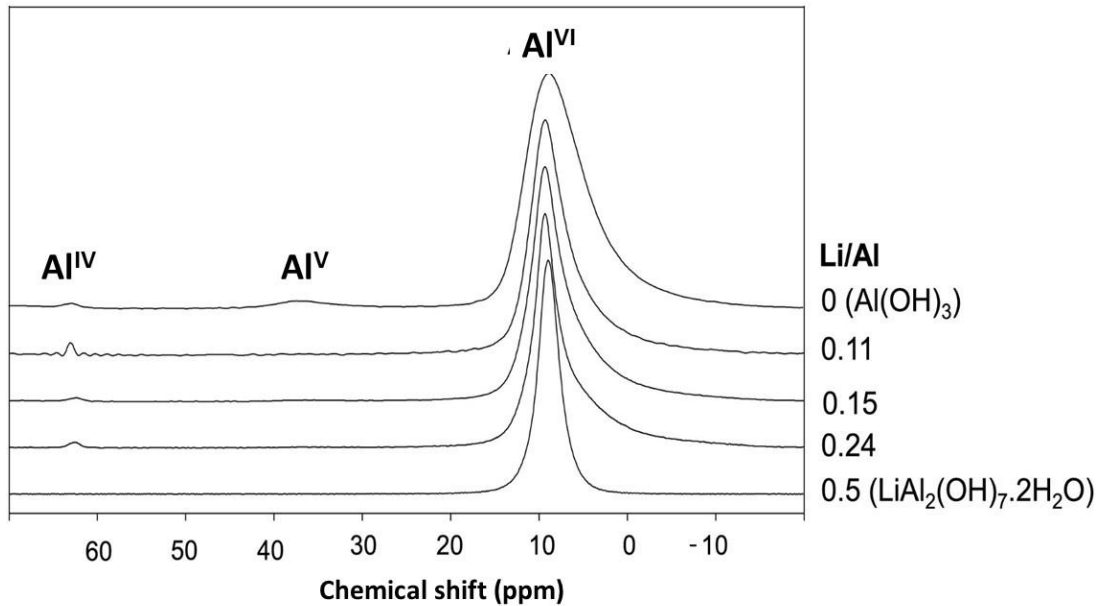
Figure 62 : spectres RMN MAS ^{27}\text{Al} (18,8 T) de \text{Al}(\text{OH})_3 mis en présence de sels de Li et en fonction du ratio molaire \text{Li}/\text{Al} , et de la phase cristalline \text{LiAl}_2(\text{OH})_7 \cdot 2\text{H}_2\text{O} .
