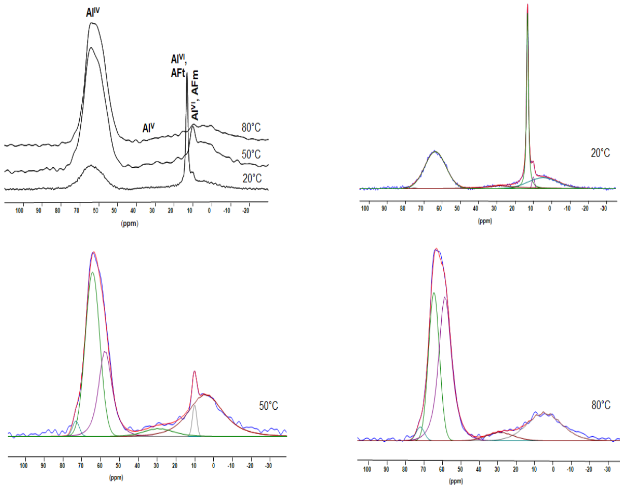
Figure 52 : spectres RMN-MAS de 27 Al (18,8 T) de la pâte B40 hydratée à 6 mois en fonction de la température de cure avec ses décompositions (AFt : Ettringite, AFm : Monosulfate). Spectre expérimental en bleu, spectre simulé en rouge.
