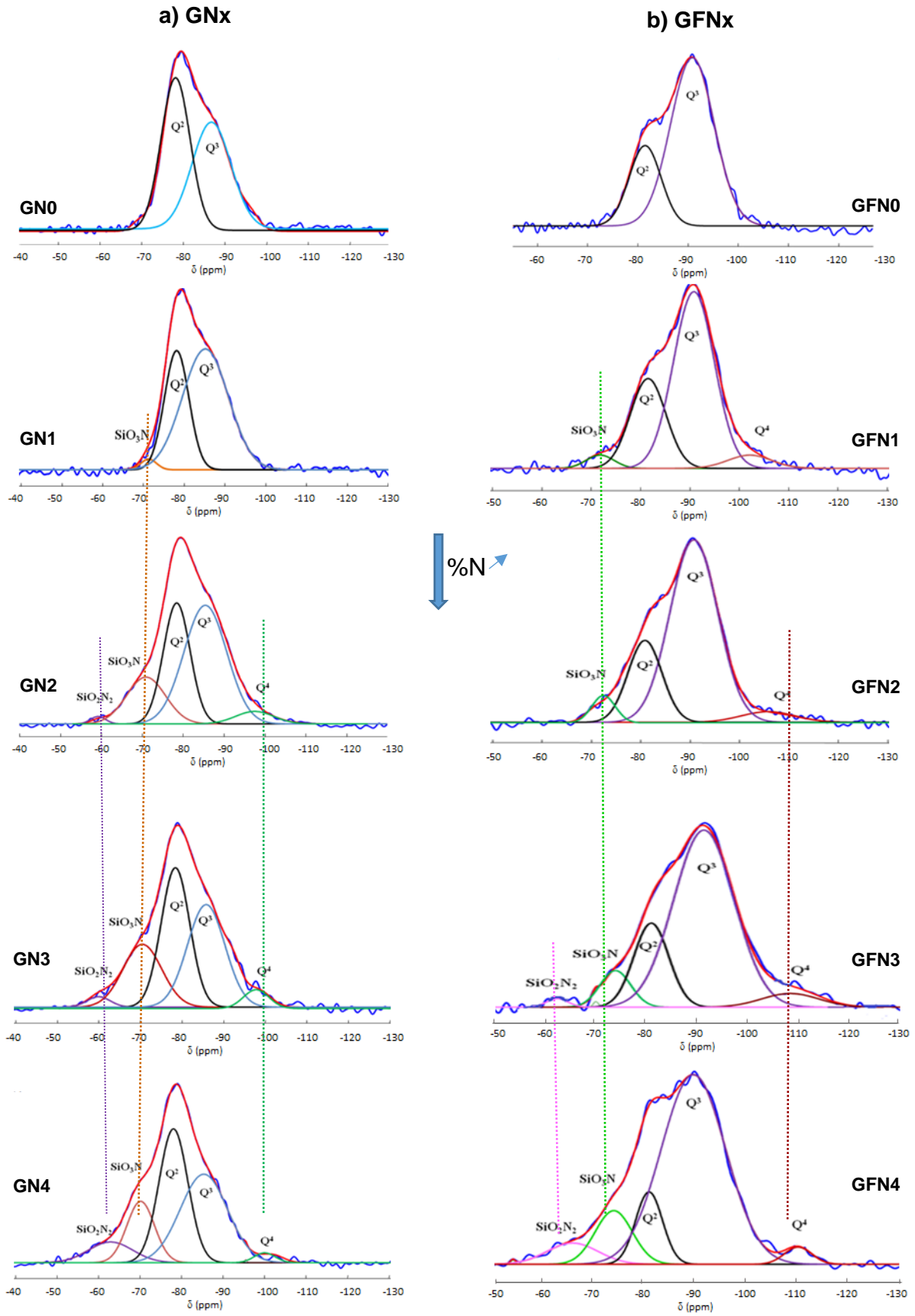
Figure 19 : spectres RMN MAS ^{29}\text{Si} des verres a) oxynitrés (GNx) et b) oxynitrés fluorés (GFNx) (9,4 T) avec leurs décompositions – Spectre expérimental en bleu, spectre simulé en rouge.
