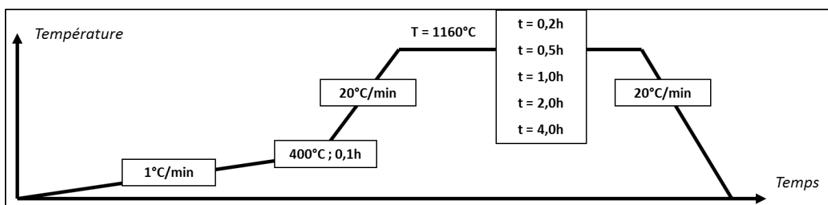
Figure 72 : Cycles de frittage – Variation de la durée de frittage
