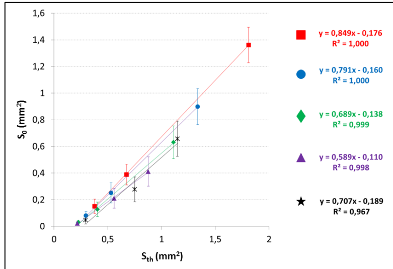
Figure 59 : Valeurs réelles des surfaces S_0 des macropores (en \text{mm}^2 ) obtenus en cru en fonction de la surface théorique S_{th} des pores sur le masque (en \text{mm}^2 )
