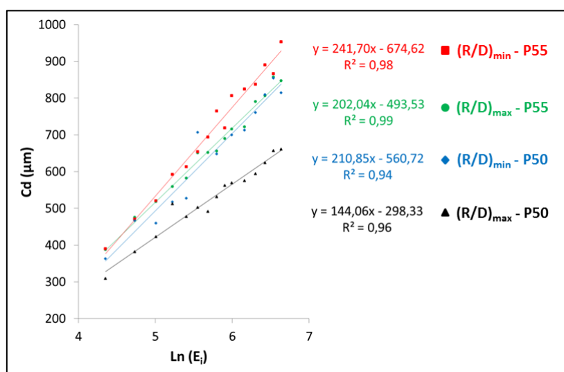
Figure 43 : Test de réactivité des suspensions passées une fois au tricylindre (épaisseurs mesurées Cd en fonction du logarithme de la densité d'énergie reçue E_i )
