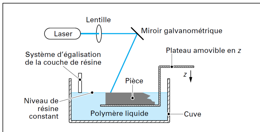
Figure 15 : Schéma de principe de stéréolithographie (BM7017 2 )
