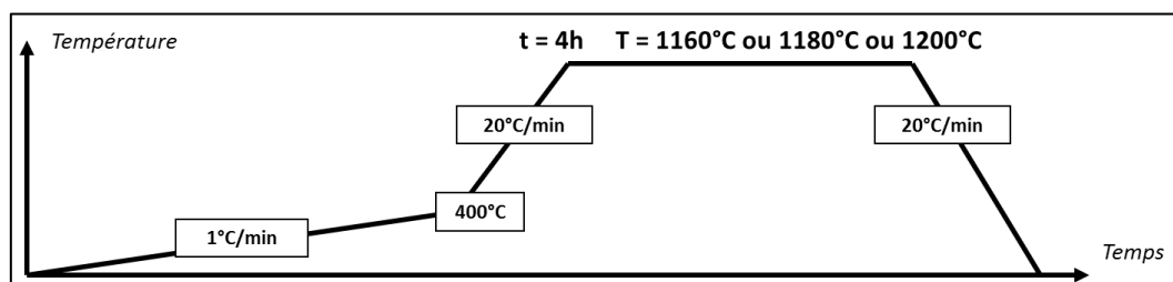
Figure 65 : Cycles thermiques suivis par dilatométrie
