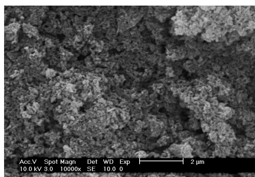
Figure 20 : Micrographie MEB de la poudre de SiHA brute
