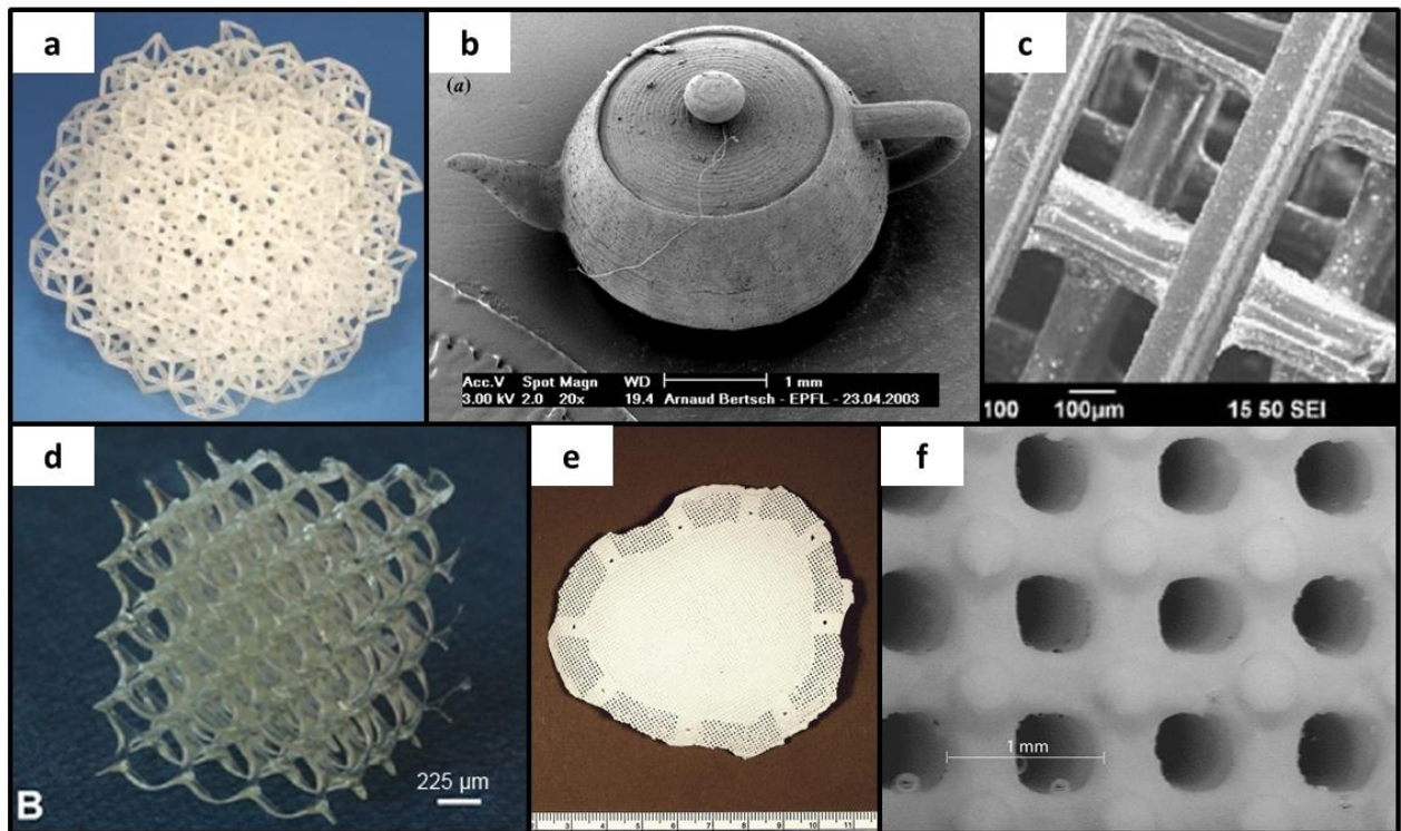
Figure 14 : Photographies et micrographies d'architectures complexes : (a) en polymère réalisée par SL par Man et al. [206], (b) en composite polymère-alumine réalisée par \mu SL par Bertsch et al. [207], (c) en composite PPF/DEF-HA réalisée par \mu SL par Lee et al. [208], (d) en polymère réalisée par \mu SL par Leigh et al. [209] ; (e) (f) en HA réalisée par \mu SL par Brie et al.[205]
