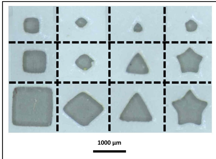
Figure 62 : Micrographies optiques de géométries macroporeuses bidimensionnelles mises en forme par microstéréolithographie, pièces en cru avant traitement thermique
