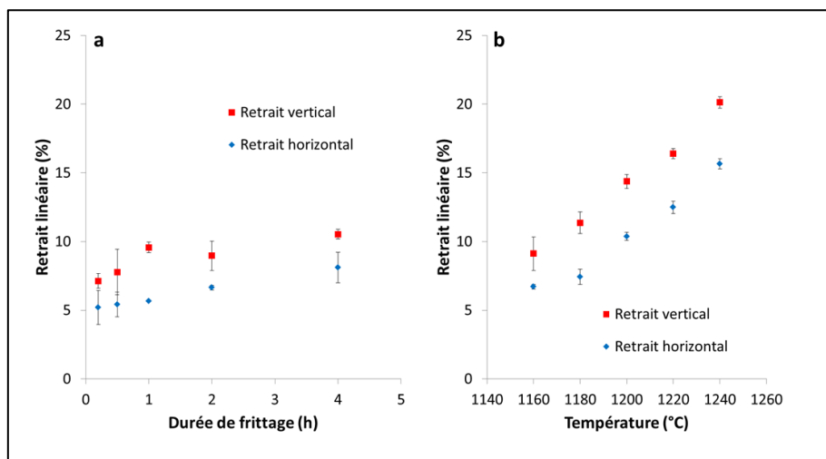
Figure 77 : Evolution du retrait linéaire avec la durée de frittage pour une température fixée à 1160°C (a) et avec la température pour une durée de frittage fixée à 2 h (b) (valeurs moyennes obtenues à partir de trois échantillons pour chaque cycle thermique)
