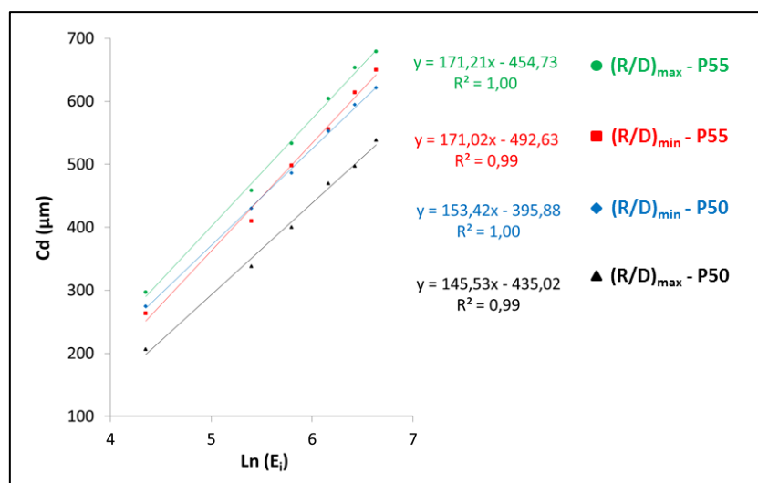
Figure 44 : Test de réactivité des suspensions passées cinq fois au tricylindre (épaisseurs mesurées C_d en fonction du logarithme de la densité d'énergie reçue E_i )
