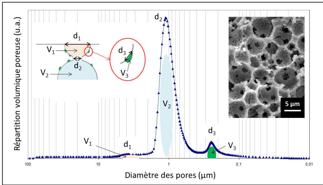
Figure 5 : Courbes de porosimétrie mercure obtenues à partir d'échantillons microporeux élaborés par hétérocoagulation [86] ( d_1 et V_1 : diamètre et volume des pores ouverts ; d_3 et V_3 : diamètre et volume des micropores présents sur les parois ; V_2 : volume des pores internes interconnectés ; d_2 : diamètre des interconnexions)
