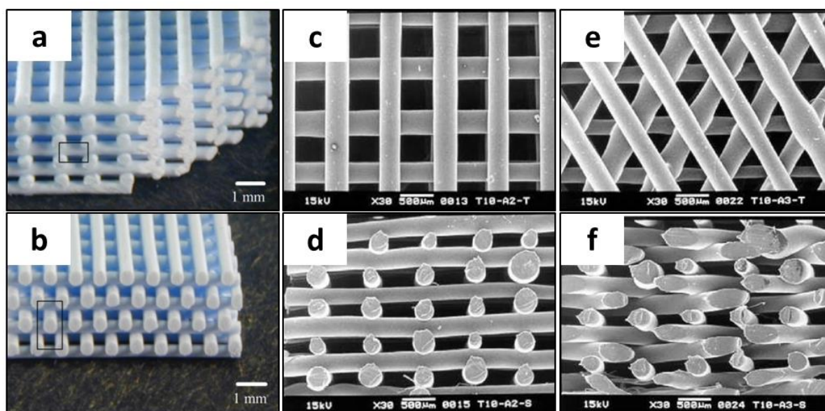
Figure 12 : Photographies et micrographies de pièces poreuses : (a) et (b) en HA réalisées par dépôt robotique par Dellinger et al. [196] ; (c) (d) (e) (f) en poly( \epsilon -caprolactone) (PCL) réalisées par dépôt robotique (FDM) par Zein et al. [193]
