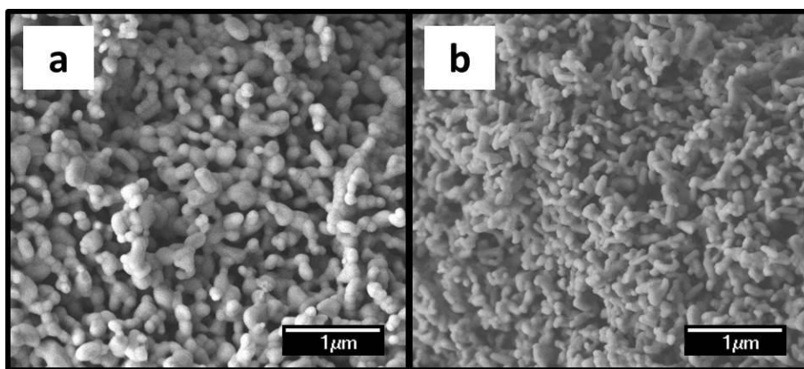
Figure 82 : Micrographies MEB des poudres HA (a) et SiHA (b), calcinées à 1000°C pendant 1 h
