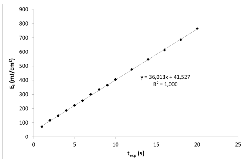
Figure 42 : Droite d'étalonnage du système d'irradiation UV (Valeurs expérimentales et régression linéaire)
