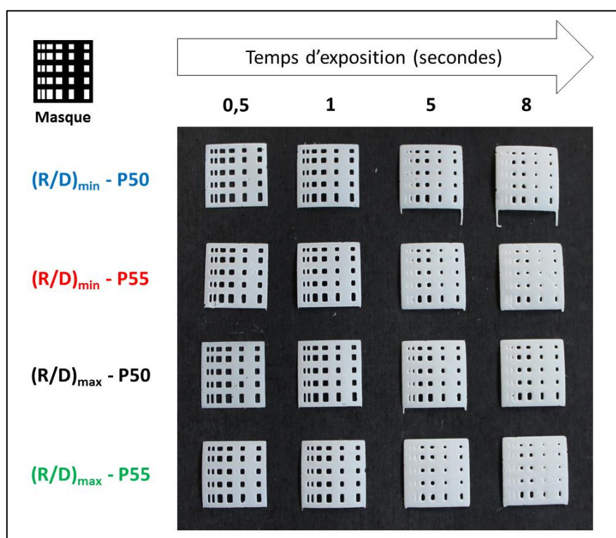
Figure 45 : Photographies des pièces monocouches réalisées avec quatre suspensions différentes et quatre temps d'exposition, à partir du même masque
