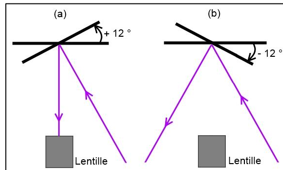
Figure 25 : Réflexion du faisceau UV sur les micromiroirs, en direction de la lentille (a) et hors du plan de travail (b)
