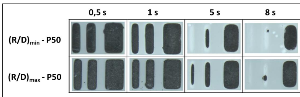
Figure 46 : Photographies de pièces mises en forme pour le test de définition : variation du ratio résine/diluant à taux de charge constant, pour différents temps d'exposition
