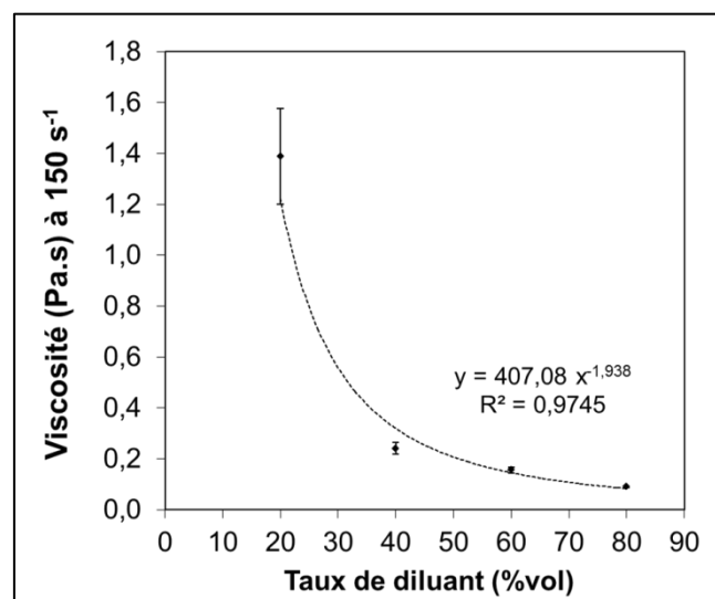
Figure 27 : Evolution de la viscosité des suspensions avec le taux de diluant (exprimé par rapport au volume total de solvant : R + D), pour un taux de charge fixé à 36 %vol
