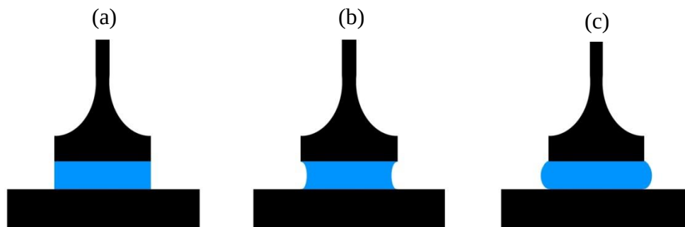
Figure 121 : Alignement de l'échantillon au cône : alignement adéquat (a), échantillon insuffisant (b), débordement (c)
