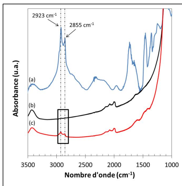
Figure 31 : Spectres IRTF du dispersant (a) et des poudres SiHA calcinées à 1200°C, non attritées (b) et attritées en présence du dispersant (c)
