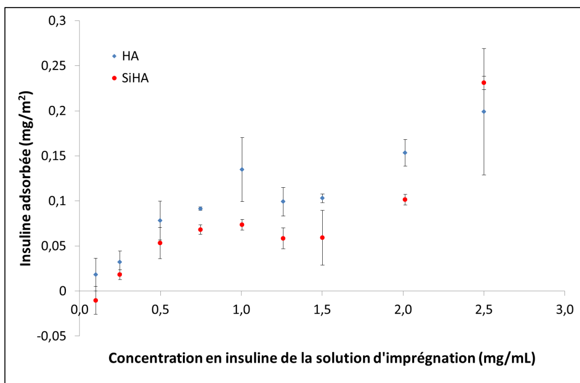
Figure 86 : Isothermes d'adsorption de l'insuline à la surface des poudres HA et SiHA calcinées à 1000°C
