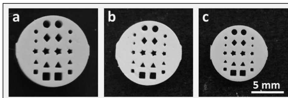
Figure 80 : Photographies de pièces de dix couches mises en forme par \mu SL : en cru (a), frittée à 1160°C – 0,2 h (b) et frittée à 1240°C – 2 h (c)
