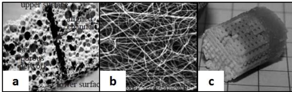
Figure 8 : Architectures poreuses : (a) aléatoire contenant un canal central [120], (b) fibreuse [122], (c) empilement de tiges parallèles à section quadratique [121]
