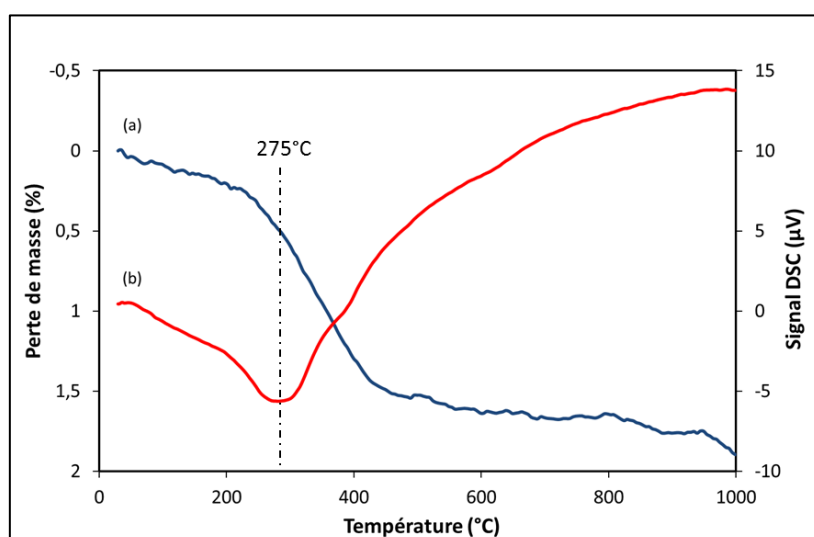
Figure 33 : Courbes d'analyse thermogravimétrique (a) et calorimétrique différentielle (b) des poudres SiHA attritées en présence de dispersant
