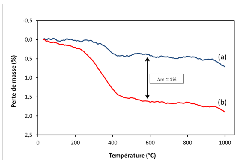
Figure 32 : Courbes d'analyse thermogravimétrique des poudres SiHA non attritées (a) et attritées en présence de dispersant (b)
