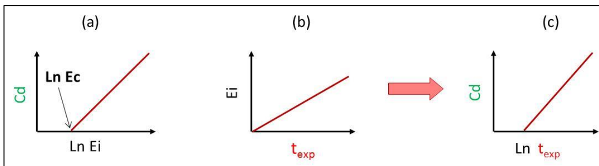
Figure 38 : Allures théoriques des représentations graphiques de l'équation de Jacobs (a), de la droite d'étalonnage (b) et du test de réactivité (c)
