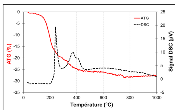
Figure 64 : Courbes d'analyse thermogravimétrique (ATG) et de signal DSC d'un échantillon mis en forme par microstéréolithographie
