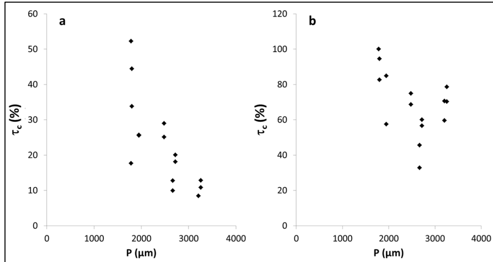
Figure 105 : Valeurs des taux de recouvrement \tau_c , après 7 jours (a) et 14 jours (b) de culture, en fonction des valeurs de périmètre P des sections des pores déterminées à partir des micrographies
