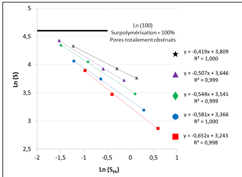
Figure 56 : Evolution de la surpolymérisation S d'un pore d'une pièce crue monocouche en fonction de la surface théorique S_{th} du pore selon le masque, pour cinq géométries de pores (transformée logarithmique)
