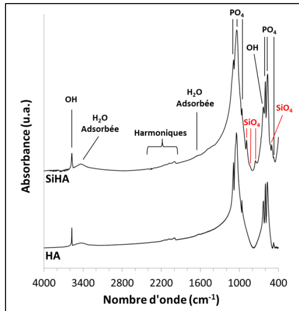
Figure 18 : Spectres infrarouge de poudres HA et SiHA calcinées à 1000°C pendant 15 h
