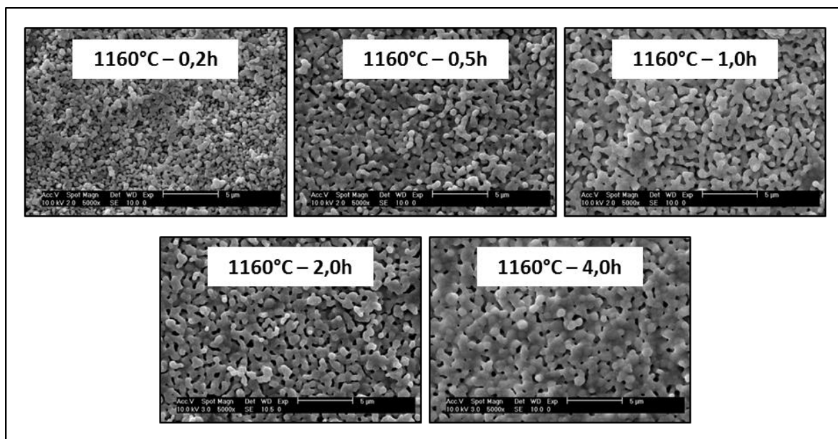
Figure 75 : Micrographies MEB d'échantillons frittés à 1160°C avec différents paliers selon les cycles présentés en Figure 72
