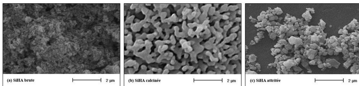
Figure 29 : Micrographies MEB de poudres de SiHA : brute (a), calcinée à 1200^\circ\text{C} - 30min (b) et attritée à 800 tr/min – 8h (c)
