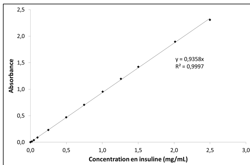
Figure 85 : Droite d'étalonnage de l'absorbance établie avec les solutions d'insuline
