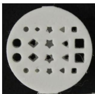
Figure 51 : Photographie d'une pièce crue de 5 couches, vue de dessus, réalisée par microstéréolithographie avec un temps d'exposition de 0,83 s et une épaisseur de suspension étalée réduite pour une couche, conduisant à l'obstruction partielle des macropores
