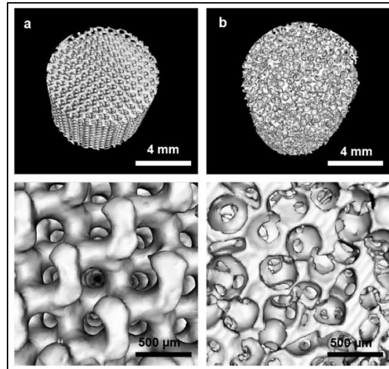
Figure 6 : Observations par microtomographie de substituts de PDLLA d'architecture gyroïde réalisée par stéréolithographie (a) et d'architecture aléatoire réalisée par lixiviation (b), Melchels et al. [116]
