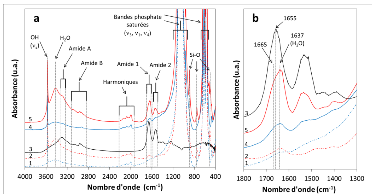
Figure 87 : Spectres IRTF de HA (ligne pointillée 1), de SiHA (ligne pointillée 2), de l'insuline (ligne pleine 3), de HAINS (ligne pleine 4) et de SiHAINS (ligne pleine 5). (a) Spectre large sur 4000 – 400 cm -1 , (b) Zoom sur la région spectrale de l'amide I.
