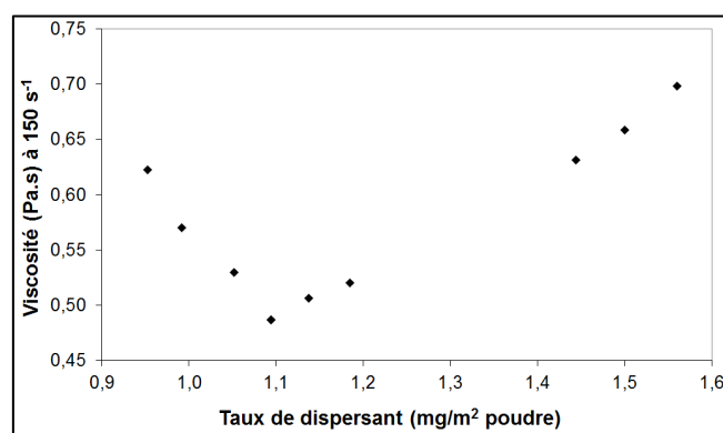
Figure 35 : Evolution de la viscosité à 150 \text{ s}^{-1} et 25^\circ\text{C} en fonction du taux de dispersant
