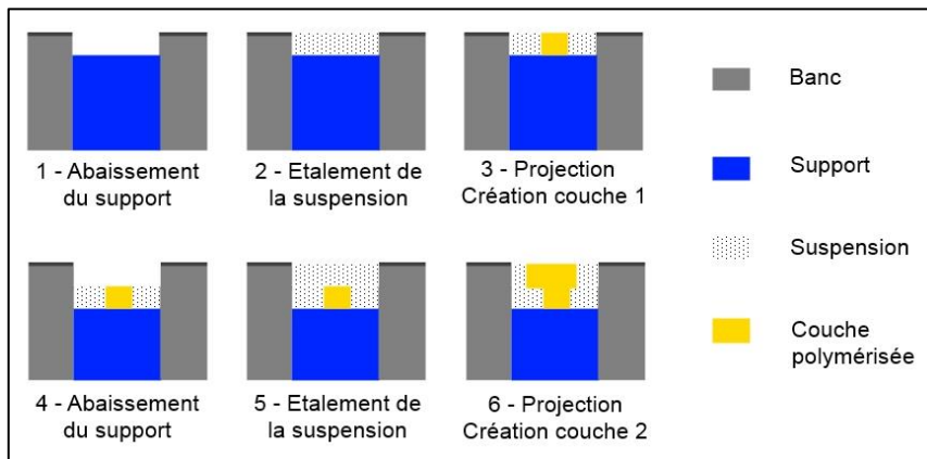
Figure 24 : Etapes de mise en forme d'une pièce 3D par microstéréolithographie (création des deux premières couches)
