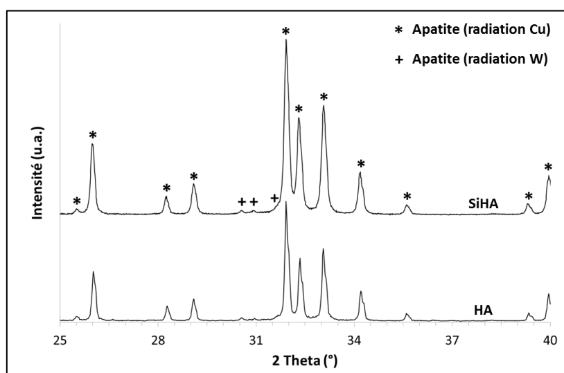
Figure 17 : Diffractogrammes de poudres HA et SiHA calcinées à 1000°C pendant 15 h, indexés selon la fiche PDF 9-432 avec les radiations du cuivre et du tungstène
