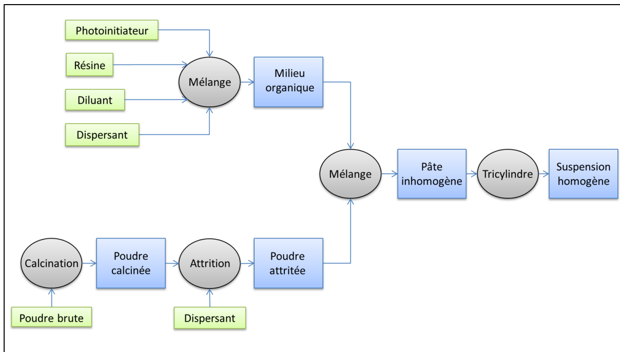
Figure 28 : Diagramme de préparation des suspensions
