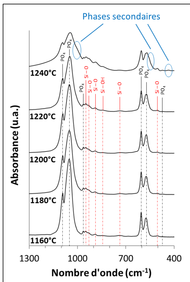
Figure 70 : Spectres IRTF des échantillons frittés respectivement à 1160°C, 1180°C, 1200°C, 1220°C et 1240°C, pendant 2 h
