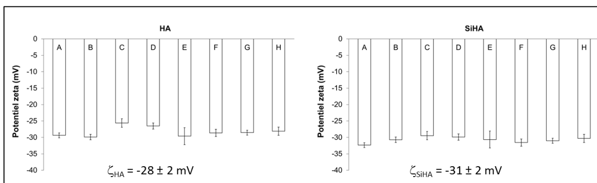
Figure 83 : Valeurs de potentiel zeta obtenues sur 8 séries (notées A à H) de 5 mesures, sur la surface de poudres d'HA et SiHA calcinées à 1000°C pendant 1 h
