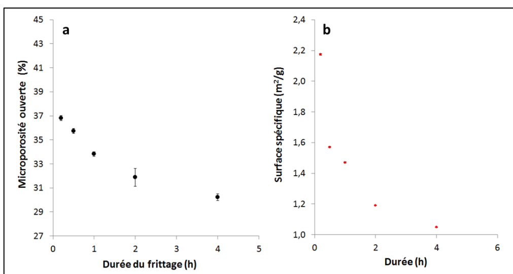
Figure 73 : Taux de microporosité ouverte (mesurés par méthode d'Archimède, moyennés sur 3 échantillons) (a) et surfaces spécifiques (mesurées par méthode BET, moyennées sur 2 échantillons) (b), en fonction de la durée de frittage, pour une température de frittage de 1160°C
