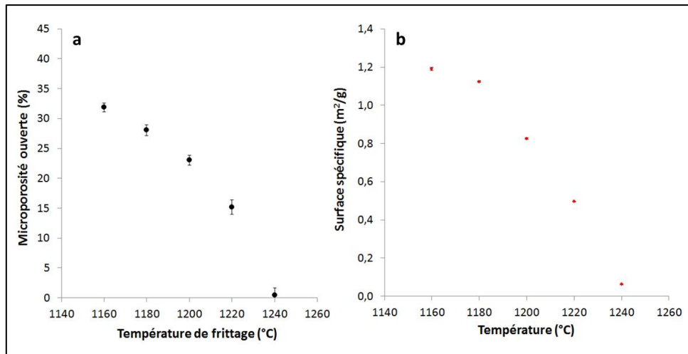
Figure 71 : Taux de microporosité ouverte (mesurés par méthode d'Archimède, moyennés sur 3 échantillons) (a) et surfaces spécifiques (mesurées par méthode BET, moyennées sur 2 échantillons)(b), en fonction des températures de frittage, pour une durée de frittage de 2 h
