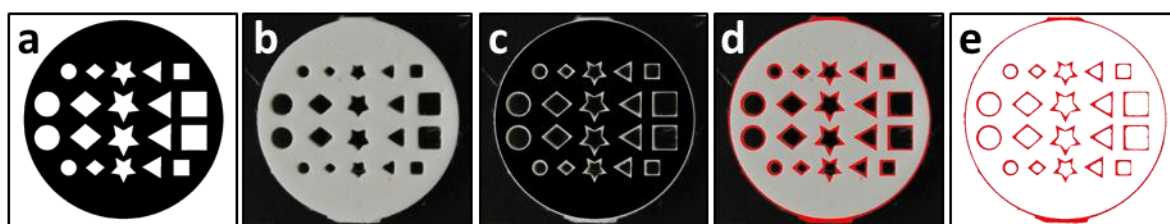
Figure 53 : Détection de la surpolymérisation par traitement d'image : a) image du masque (calque M), b) image de la pièce, c) superposition du calque M sur l'image de la pièce, d) coloration en rouge de la zone surpolymérisée sur la pièce, e) calque S
