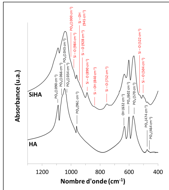
Figure 19 : Spectres infrarouge de poudres HA et SiHA calcinées à 1000°C pendant 15 h, agrandissement sur la zone spectrale 400-1300 \text{cm}^{-1} (les indexations représentées en noir sont communes aux spectres d'HA et SiHA, les indexations représentées en rouge sont spécifiques aux spectres de SiHA)
