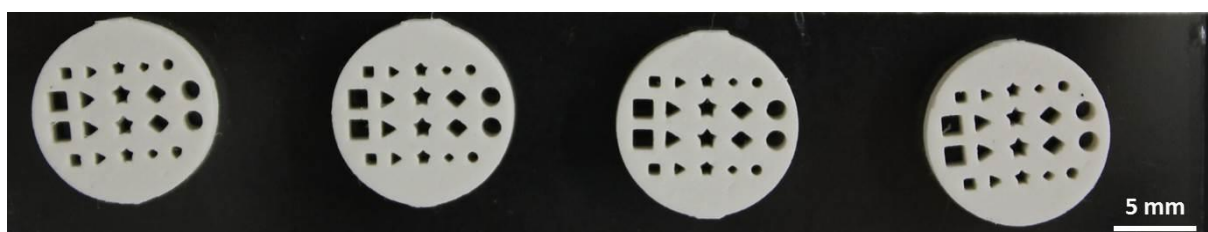
Figure 100 : Photographie de substrats de 10 couches en cru (vus de dessus)
