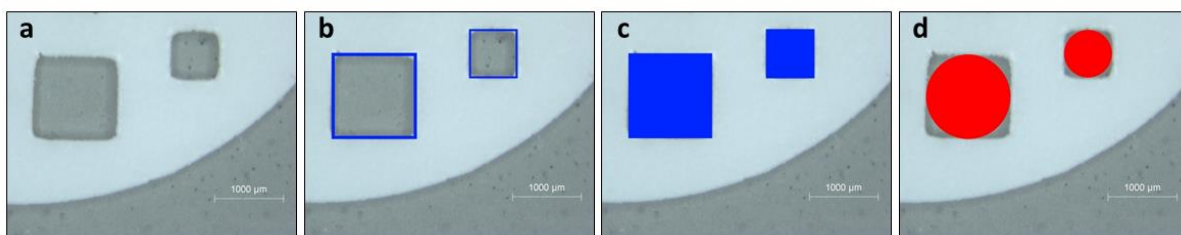
Figure 101 : Photographie d'un substrat vu de dessus (a), périmètre P (b) et surface S_0 (c) (colorés en bleu) des domaines définis par les sections horizontales des macropores ; cercles de diamètre D_i inscrits dans les géométries de ces domaines (colorés en rouge) (d)
