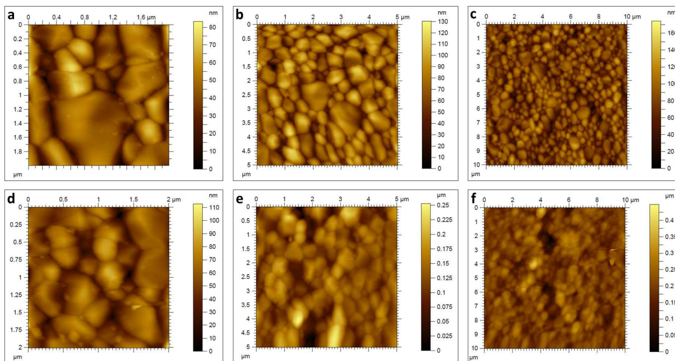
Figure 91 : Topographies AFM des pastilles HA (a, b, c) et SiHA (d, e, f), frittées à 1200°C pendant 1 h, non polies
