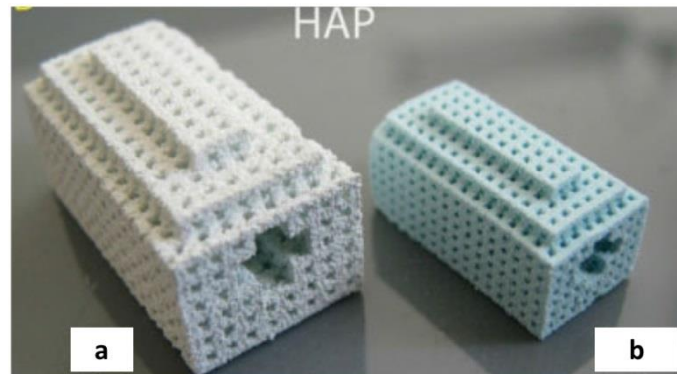
Figure 13 : Photographie de pièces poreuses en HA réalisées par 3DP par Warnke et al. [199] avant (a) puis après (b) frittage
