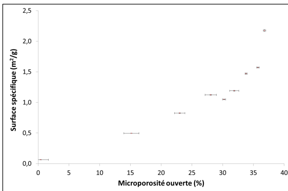
Figure 74 : Valeurs de surface spécifique (mesurées par méthode BET, moyennées sur deux échantillons) en fonction des taux de microporosité ouverte (mesurés par méthode d'Archimède, moyennés sur trois échantillons)
