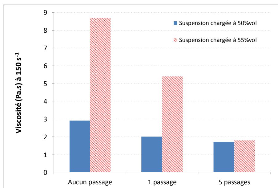
Figure 34 : Evolution de la viscosité des suspensions avec les passages au tricylindre
