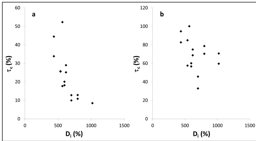
Figure 107 : Valeurs des taux de recouvrement \tau_c , après 7 jours (a) et 14 jours (b) de culture, en fonction du diamètre D_i des cercles inscrits dans les pores déterminé à partir des micrographies
