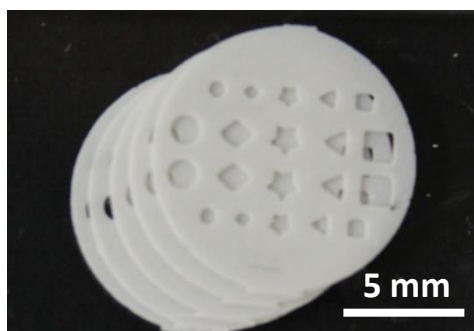
Figure 50 : Photographie d'une pièce crue de 5 couches, vue de dessus, réalisée par microstéréolithographie avec un temps d'exposition de 0,83 s et une épaisseur de suspension étalée de 255 \mu\text{m} (couches non adhérentes)
