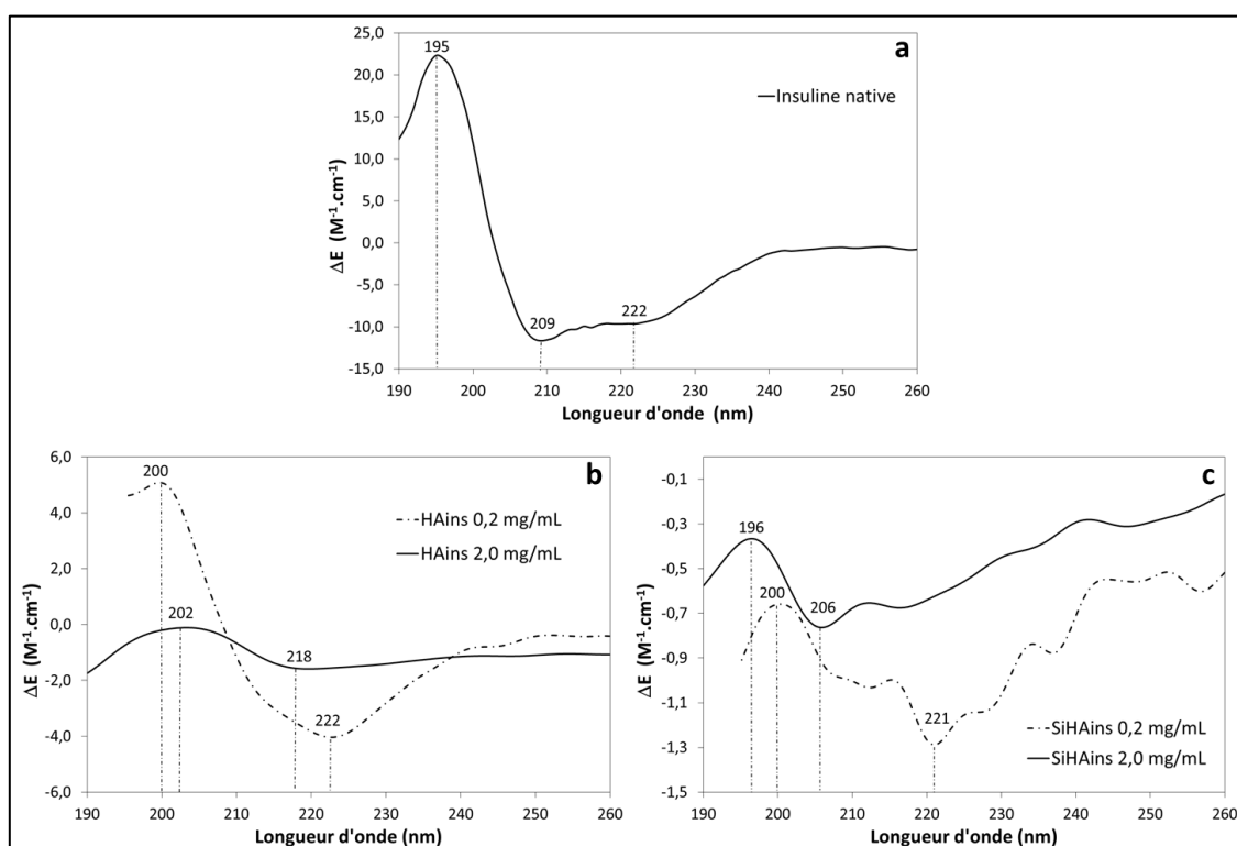
Figure 88 : Spectres CD de (a) l'insuline native, (b) l'insuline adsorbée sur la poudre d'HA : HAins 0,2 mg/mL et HAins 2,0 mg/mL, (c) l'insuline adsorbée sur la poudre de SiHA : SiHAins 0,2 mg/mL et SiHAins 2,0 mg/mL
