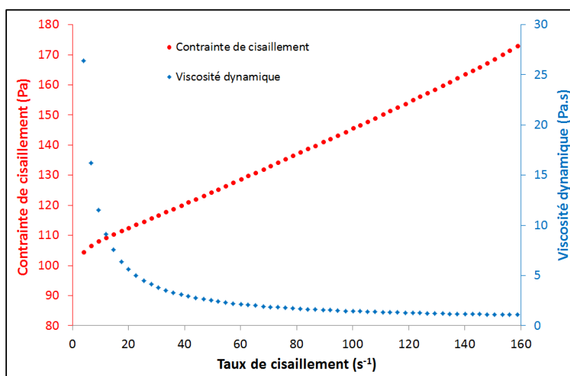
Figure 37 : Rhéogramme de la suspension (R/D)_{min}-P50 (les rhéogrammes des suspensions (R/D)_{min}-P55 , (R/D)_{max}-P50 et (R/D)_{max}-P55 sont similaires avec des valeurs de contraintes seuil et de viscosité plus élevées)
