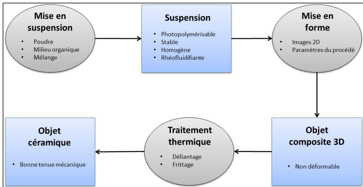
Figure 21 : Etapes de développement d'un objet céramique 3D par microstéréolithographie
