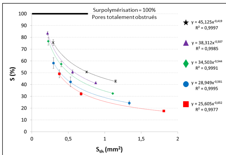
Figure 55 : Evolution de la surpolymérisation S d'un pore d'une pièce crue monocouche en fonction de la surface théorique S_{th} du pore selon le modèle du masque, pour cinq géométries de pores
