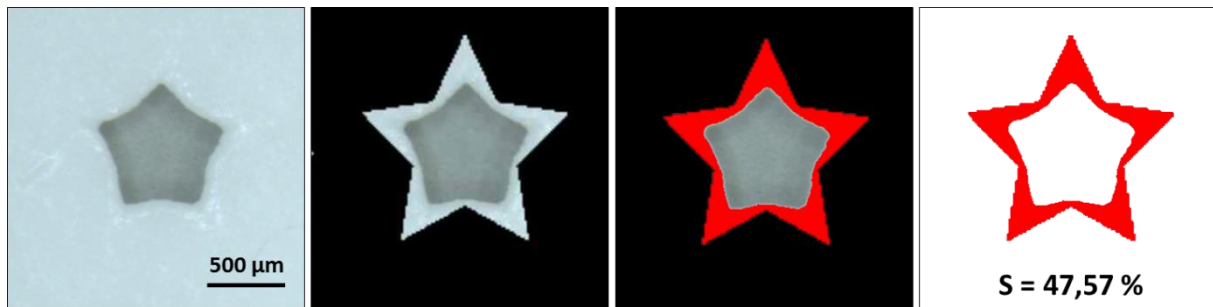
Figure 54 : Calcul de la surpolymérisation à partir de traitement d'image, pour un macropore en forme d'étoile
