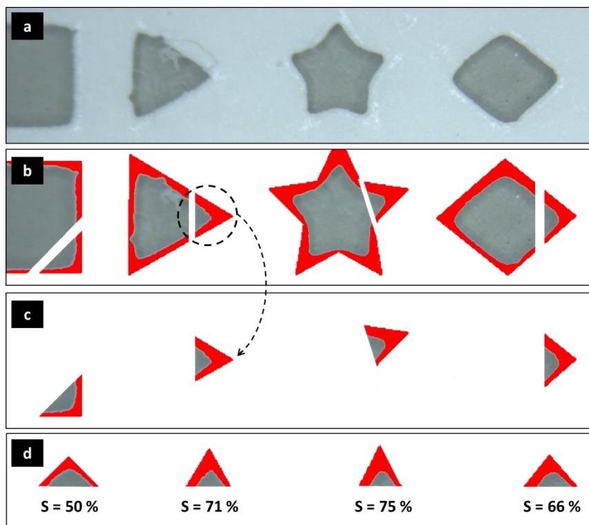
Figure 61 : Détermination de la surpolymérisation à l'intérieur des angles : photographie de la pièce (a), coloration de la surpolymérisation et découpe des angles à surface identique (b), extraction des angles de surface égale (c), calcul de la surpolymérisation dans les angles (d)
