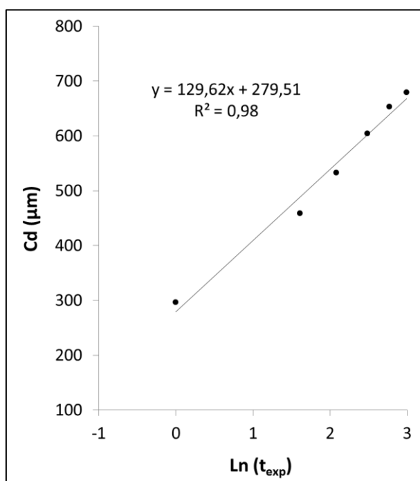
Figure 49 : Epaisseurs polymérisées Cd, reportées en fonction du logarithme du temps d'exposition t_{exp} , et régression linéaire
