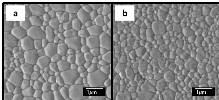
Figure 90 : Micrographies MEB des pastilles HA (a) et SiHA (b), frittées à 1200°C-1 h, et polies
