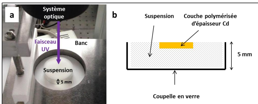
Figure 39 : Test de réactivité (a : photographie du montage ; b : schéma de la vue en tranche de la coupelle de verre contenant la suspension)
