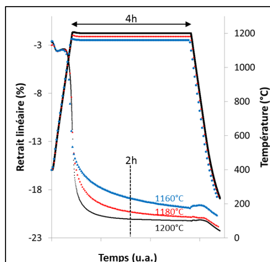
Figure 66 : Courbes de température et de retrait linéaire, en fonction du temps
