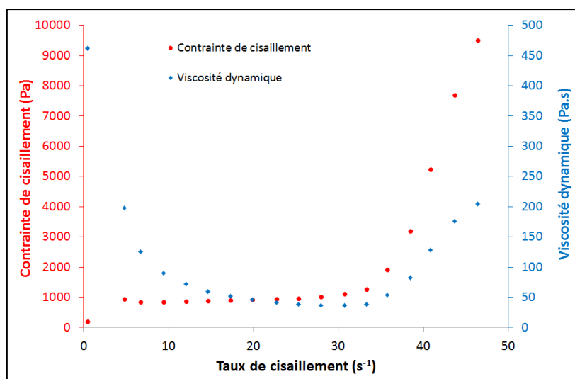
Figure 36 : Rhéogramme de la suspension (R/D)_{min}-P60
