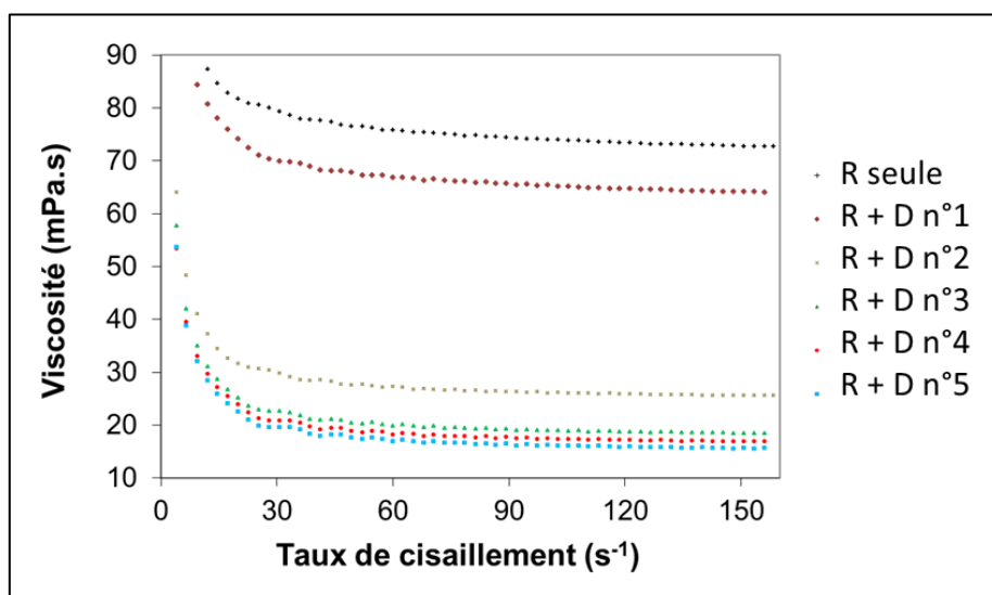
Figure 26 : Courbes d'écoulement de la résine R et des mélanges résine R – diluant D, à 25^\circ\text{C}
