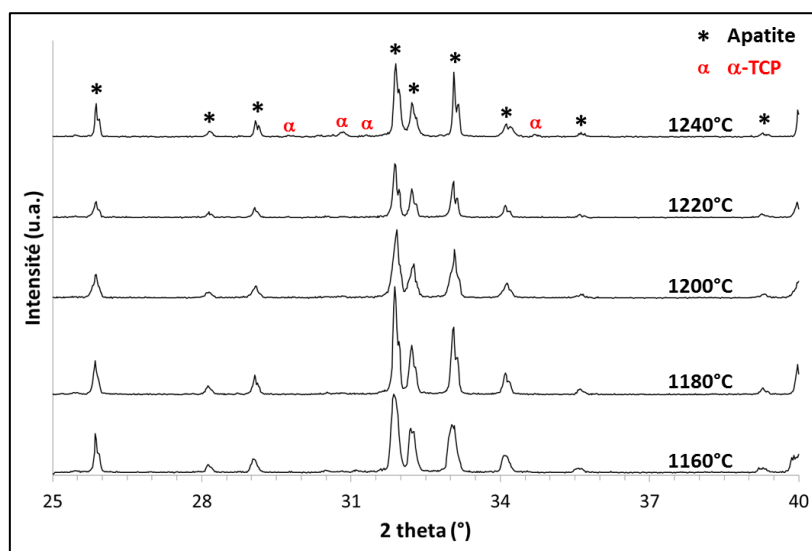
Figure 68 : Diffractogrammes des échantillons frittés respectivement à 1160°C, 1180°C, 1200°C, 1220°C et 1240°C, pendant 2h
