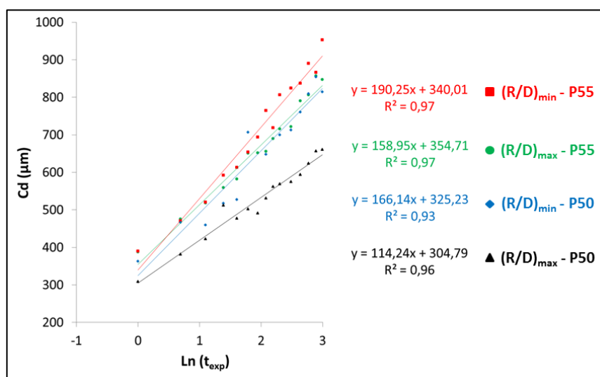
Figure 40 : Test de réactivité des suspensions passées une fois au tricylindre (épaisseurs mesurées Cd en fonction du logarithme du temps d'exposition t_{exp} )
