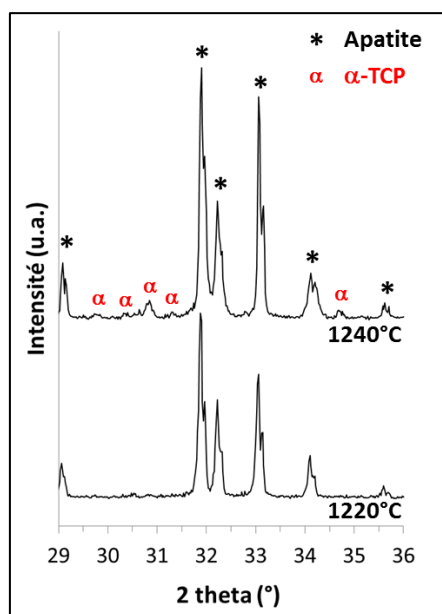
Figure 69 : Diffractogrammes des échantillons frittés respectivement à 1220°C et 1240°C, pendant 2h
