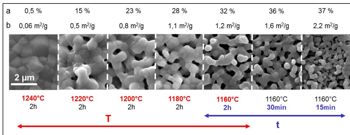
Figure 79 : Evolution du taux de microporosité ouverte (a) et de la surface spécifique (b) des échantillons SiHA mis en forme par \mu SL, en fonction des paramètres de frittage
