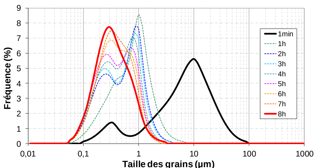
Figure 30 : Evolution de la distribution granulométrique des poudres SiHA durant l'attrition (fréquence en volume)
