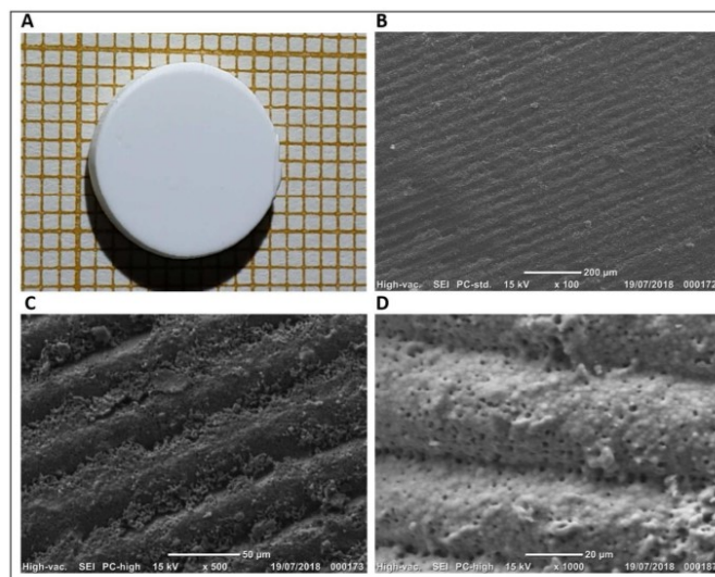
Figure 14 : A : Photo d'un  chantillon de mat riau \beta -TCP. Microscopie  lectronique   balayage (MEB) de l' tat de surface des mat riaux \beta -TCP : les vues ont  t  obtenues avec un FEG SU5000-Hitachi avec des grossissements (B) X100, (C) X500 et (D) \times 1000 apr s rev tement d'or.
